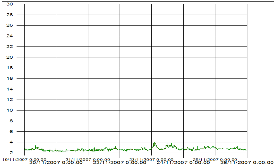
Figur 4 Turbiditet for perioden 19. - 25. november 2007 ved referansestasjonen ved serviceflåten i Bestumkilen under mudring i Bestumkilen. Y-aksen angir målt turbiditet (NTU).
