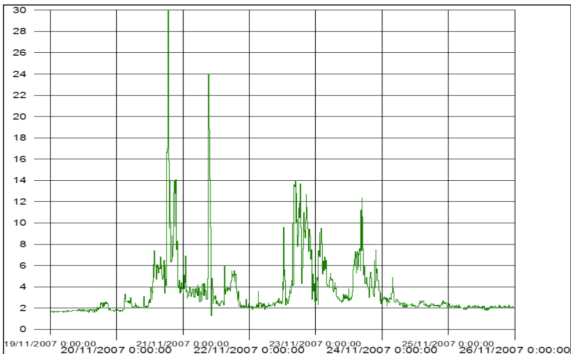
Figur 3 Turbiditet for perioden 19. - 25. november 2007 ved mudringsleker i Bestumkilen. Y-aksen angir målt turbiditet (NTU). Alle stopp som følge av overskredet grenseverdi for turbiditet blir dokumentert i månedsrapport for november.
