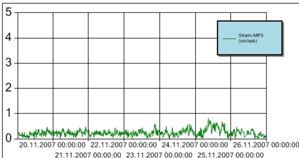
Figur 14 Strømhastighet for perioden 19. - 25. november 2007 ved målestasjon MP3. Y-aksen angir strømhastighet i cm/sekund. Sensoren er forankret slik at den henger fritt ca. 3 m over sjøbunnen.
