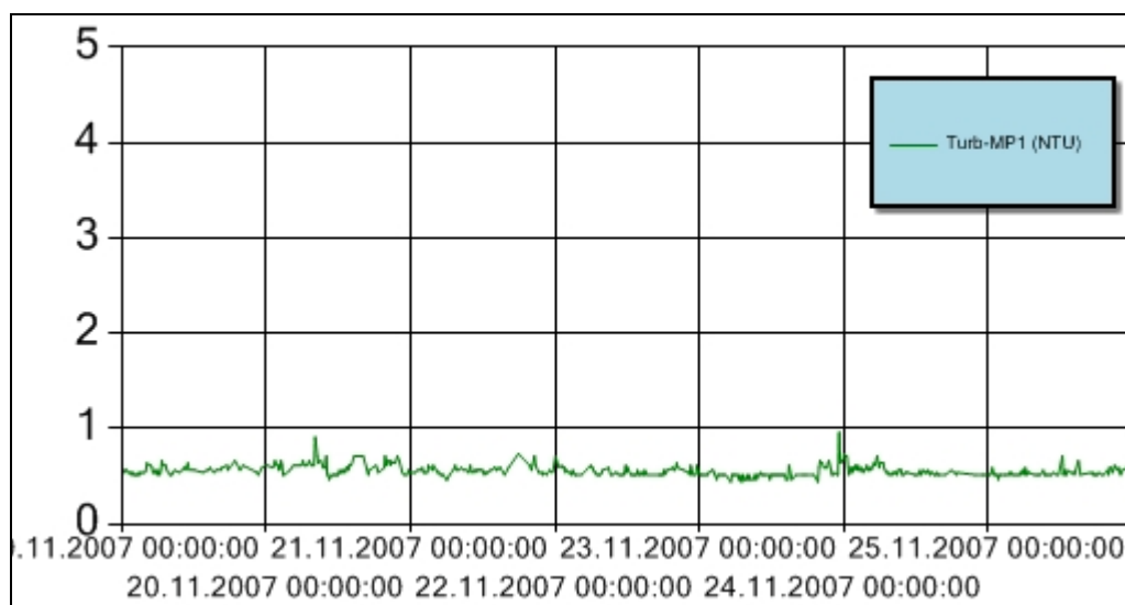
Figur 6 Turbiditet for perioden 19. - 25. november 2007 ved målestasjon MP1. Y-aksen angir målt turbiditet (NTU). Turbiditetsensoren er plassert ca. 3 m over sjøbunnen.
