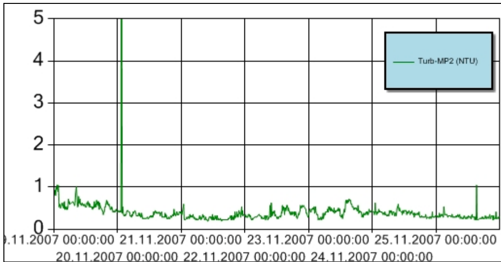
Figur 7 Turbiditet for perioden 19. - 25. november 2007 ved målestasjon MP2. Y-aksen angir målt turbiditet (NTU). Turbiditetsensoren er plassert ca. 3 m over sjøbunnen. Høye enkeltmålinger skyldes støy.
