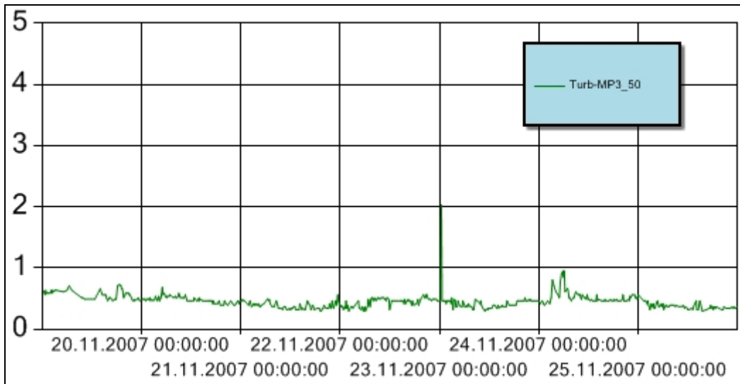
Figur 9 Turbiditet for perioden 19. - 25. november 2007 ved målestasjon MP3_50. Y-aksen angir målt turbiditet (NTU). Turbiditetsensoren er plassert ved 50 m vanddyb.
