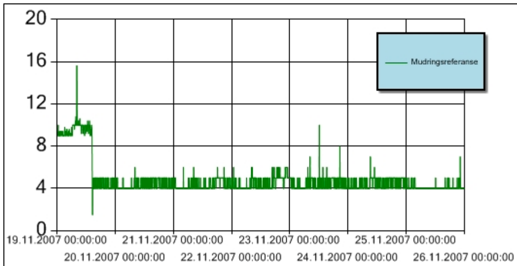
Figur 2 Turbiditet for perioden 19. - 25. november 2007 ved referansestasjonen ved Akershusutstikkeren under mudring i Pipervika. Y-aksen angir målt turbiditet (NTU). Høye enkeltmålinger skyldes støy.
