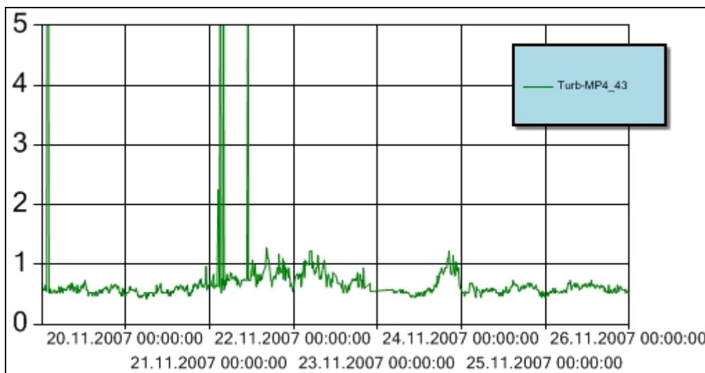
Figur 12 Turbiditet for perioden 19. - 25. november 2007 ved målestasjon MP4_43. Y-aksen angir målt turbiditet (NTU). Turbiditetsensoren er plassert ved 43 m vann dybde. Høye enkeltmålinger skyldes støy.
