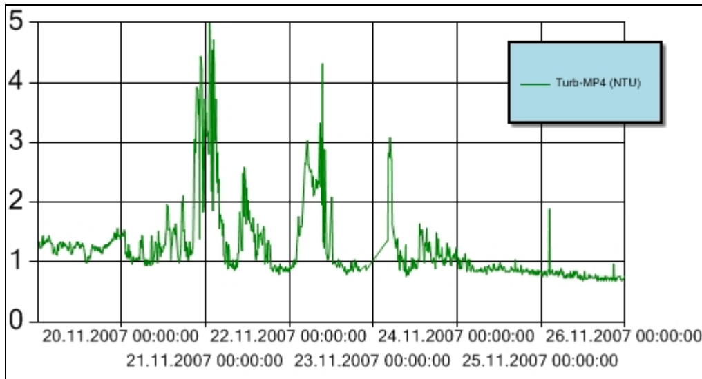
Figur 11 Turbiditet for perioden 19. - 25. november 2007 ved målestasjon MP4. Y-aksen angir målt turbiditet (NTU). Turbiditetsensoren er plassert ca. 3 m over sjøbunnen.
