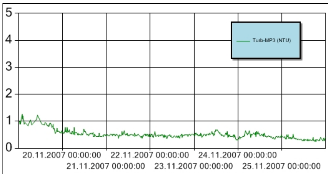
Figur 8 Turbiditet for perioden 19. - 25. november 2007 ved målestasjon MP3. Y-aksen angir målt turbiditet (NTU). Turbiditetsensoren er plassert ca. 3 m over sjøbunnen.
