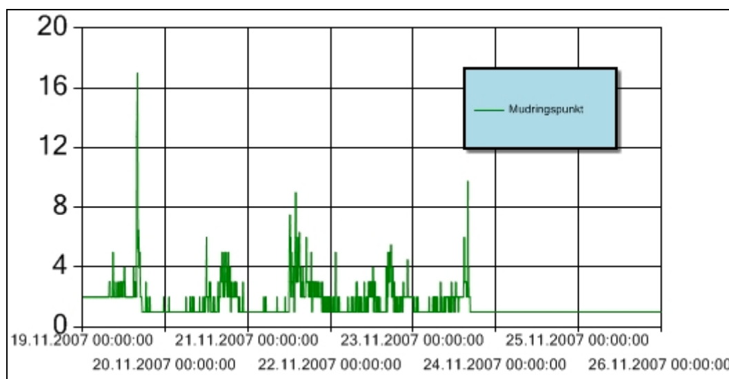
Figur 1 Turbiditet for perioden 19. - 25. november 2007 ved mudringslekter under mudring i Pipervika. Y-aksen angir målt turbiditet (NTU). Alle stopp som følge av overskredet grenseverdi for turbiditet blir dokumentert i månedsrapport for november. Høye enkeltmålinger skyldes støy.
