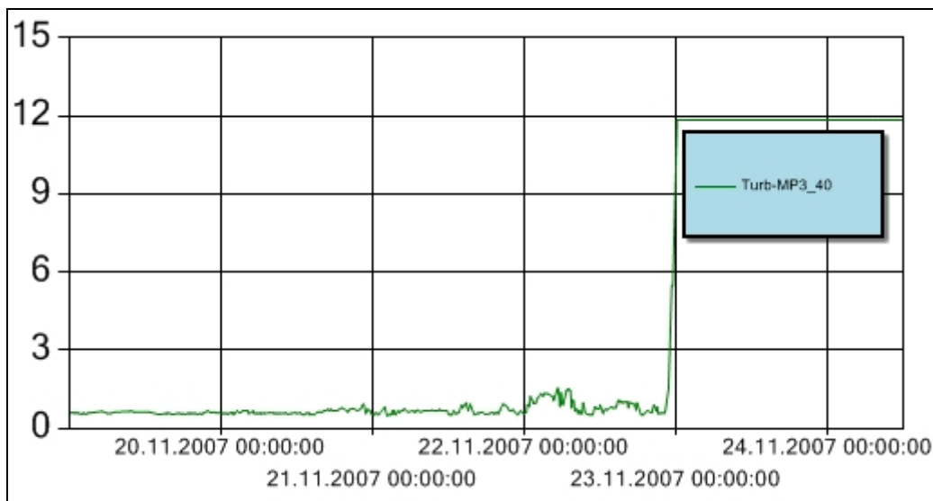
Figur 10 Turbiditet for perioden 19. - 25. november 2007 ved målestasjon MP3_40. Y-aksen angir målt turbiditet (NTU). Turbiditetsensoren er plassert ved 40 m vanddyb. Merk at MP3_40 er oppgitt med en annen skala enn de andre målerne. Den 23. november sluttet måleren å sende reelle data.
