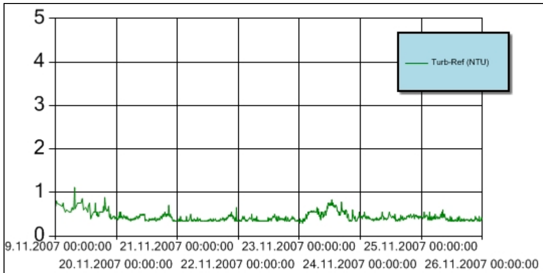
Figur 13 Turbiditet for perioden 19. - 25. november 2007 ved referansestasjonen i Bekkelagsbassenget. Turbiditetsensoren er plassert ca. 3 m over sjøbunnen. Y-aksen angir målt turbiditet (NTU).
