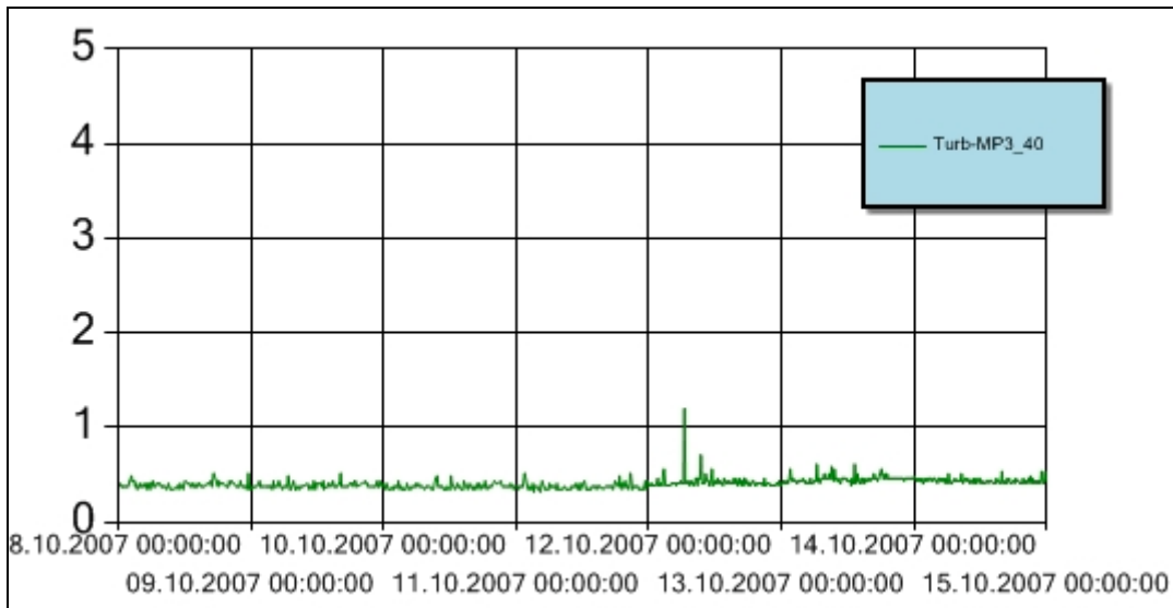
Figur 10 Turbiditet for perioden 8. – 14. oktober 2007 ved målestasjon MP3_40. Y-aksen angir målt turbiditet (NTU). Turbiditetsensoren er plassert ved 40 m vanddyb.
