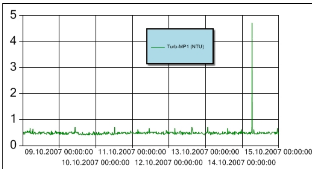
Figur 6 Turbiditet for perioden 8. – 14. oktober 2007 ved målestasjon MP1. Y-aksen angir målt turbiditet (NTU). Turbiditetsensoren er plassert ca. 3 m over sjøbunnen. Høye enkeltmålinger skyldes støy.
