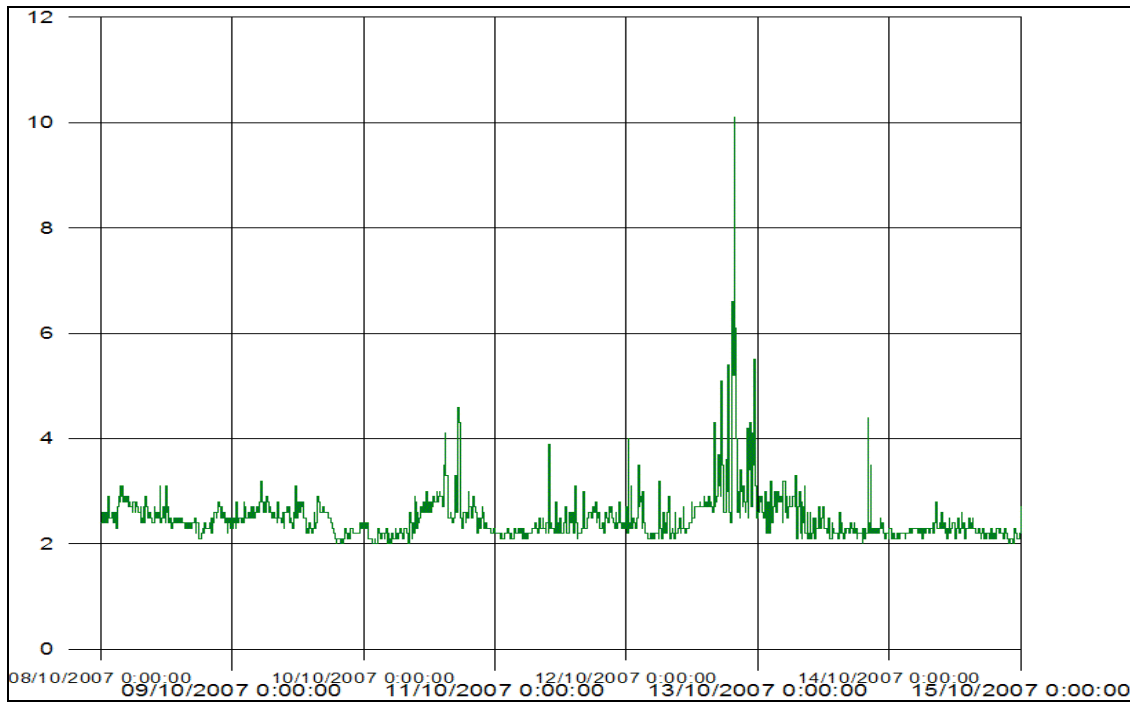
Figur 4 Turbiditet for perioden 8. – 14. oktober 2007 ved referansestasjonen ved serviceflåten i Bestumkilen under mudring i Bestumkilen. Y-aksen angir målt turbiditet (NTU). Høye enkeltmålinger skyldes støy.
