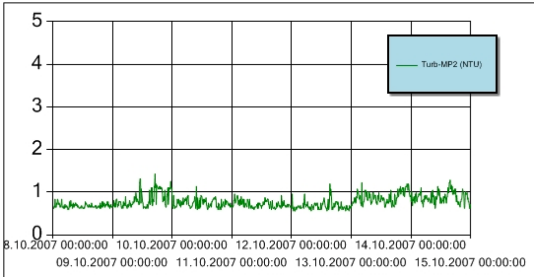
Figur 7 Turbiditet for perioden 8. – 14. oktober 2007 ved målestasjon MP2. Y-aksen angir målt turbiditet (NTU). Turbiditetsensoren er plassert ca. 3 m over sjøbunnen.
