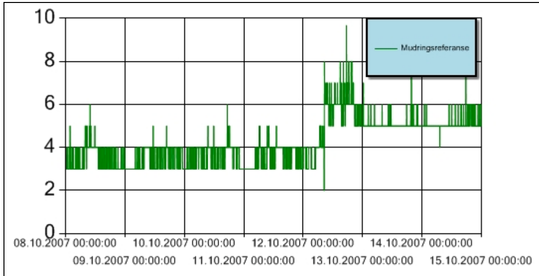
Figur 2 Turbiditet for perioden 8. – 14. oktober 2007 ved referansestasjonen ved Sørengutstikkeren under mudring i Lohavn. Y-aksen angir målt turbiditet (NTU). Høye enkeltmålinger skyldes støy.
