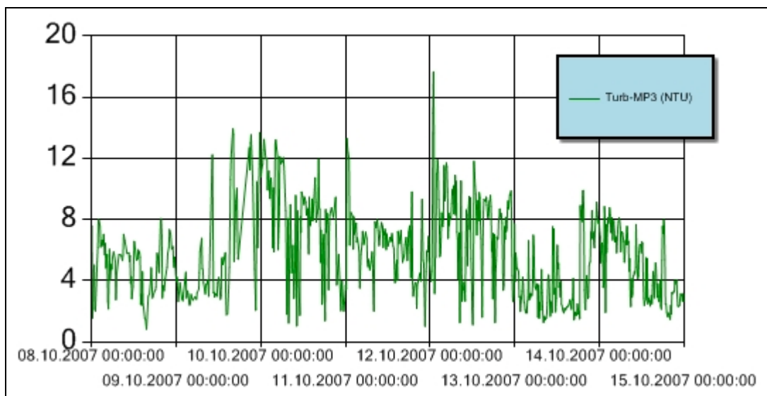
Figur 8 Turbiditet for perioden 8. – 14. oktober 2007 ved målestasjon MP3. Y-aksen angir målt turbiditet (NTU). Turbiditetsensoren er plassert ca. 3 m over sjøbunnen. Merk at MP3 er oppgitt med en annen skala enn de andre målerne.
