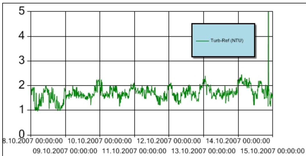
Figur 13 Turbiditet for perioden 8. – 14. oktober 2007 ved referansestasjonen i Bekkelagsbassenget. Turbiditetsensoren er plassert ca. 3 m over sjøbunnen. Y-aksen angir målt turbiditet (NTU). Høye enkeltverdier skyldes støy.
