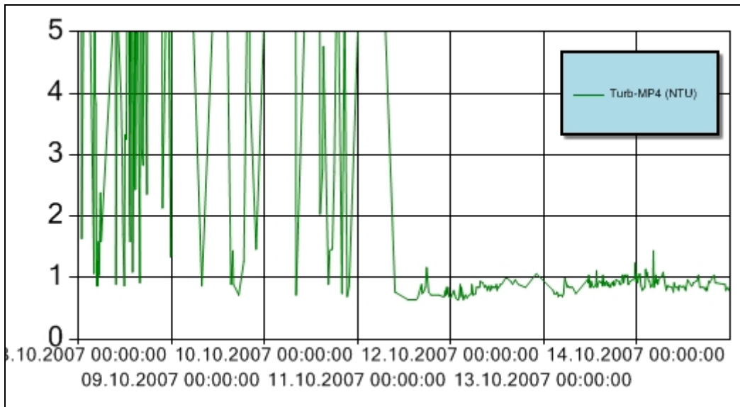
Figur 11 Turbiditet for perioden 8. – 14. oktober 2007 ved målestasjon MP4. Y-aksen angir målt turbiditet (NTU). Turbiditetsensoren er plassert ca. 3 m over sjøbunnen. Bøyen har slitt seg, og data fra uke 41 blir ikke benyttet i statistiske beregninger, fordi bøyen ligger forføyd i MPI og den nederste måleren ligger på bunnen.
