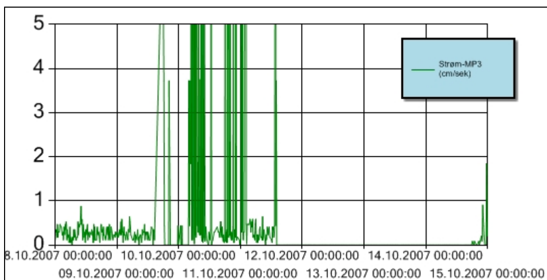
Figur 14 Strømhastighet for perioden 8. – 14. oktober 2007 ved målestasjon MP3. Y-aksen angir strømhastighet i cm/sekund. Sensoren er forankret slik at den henger fritt ca. 3 m over sjøbunnen. Det har vært en del uregelmessigheter ved måleren og data fra 9. oktober kl. 1746 – 10. oktober kl. 0955 og 11. oktober kl. 1325 – 14. oktober kl. 2136 har blitt tatt ut av de statistiske beregningene.
