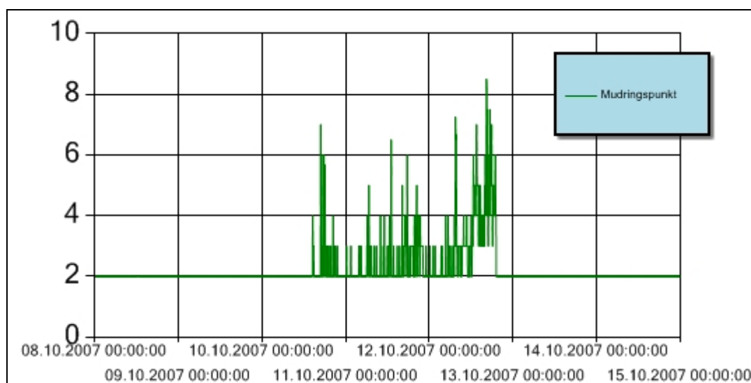
Figur 1 Turbiditet for perioden 8. – 14. oktober 2007 ved mudringslekter under mudring i Lohavn. Y-aksen angir målt turbiditet (NTU). Alle stopp som følge av overskredet grenseverdi for turbiditet blir dokumentert i månedsrapport for oktober.
