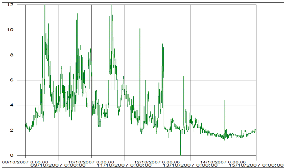
Figur 3 Turbiditet for perioden 8. – 14. oktober 2007 ved mudringslekter i Bestumkilen. Y-aksen angir målt turbiditet (NTU). Alle stopp som følge av overskredet grenseverdi for turbiditet blir dokumentert i månedsrapport for oktober.
