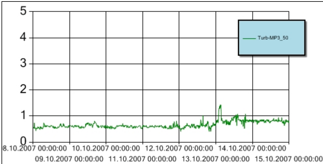
Figur 9 Turbiditet for perioden 8. – 14. oktober 2007 ved målestasjon MP3_50. Y-aksen angir målt turbiditet (NTU). Turbiditetsensoren er plassert ved 50 m vanddyb.
