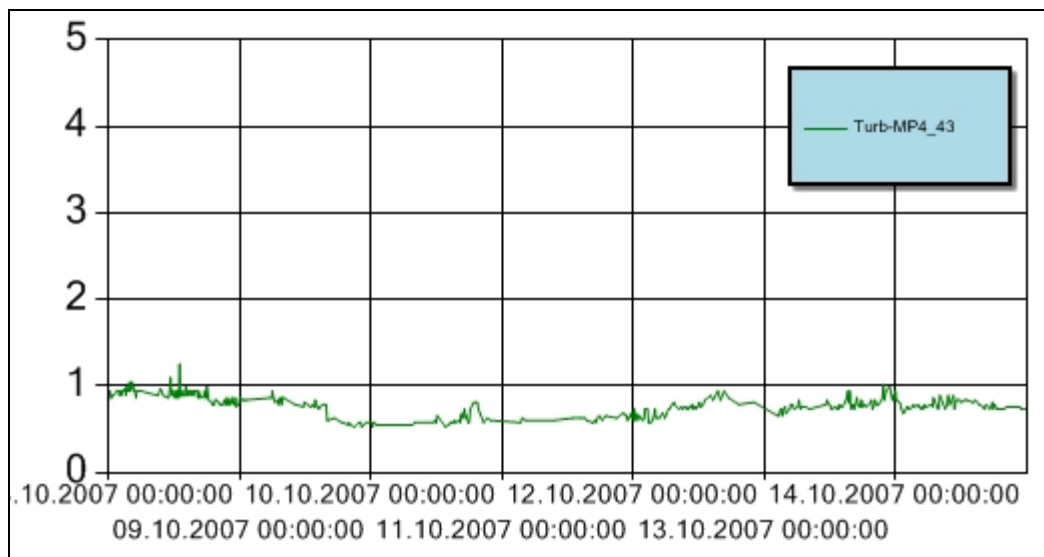
Figur 12 Turbiditet for perioden 8. – 14. oktober 2007 ved målestasjon MP4_43. Y-aksen angir målt turbiditet (NTU). Turbiditetsensoren er plassert ved 43 m vann dybde. Bøyen har slitt seg, og data fra uke 41 blir ikke benyttet i statistiske beregninger, fordi bøyen ligger forføyd i MPI.
