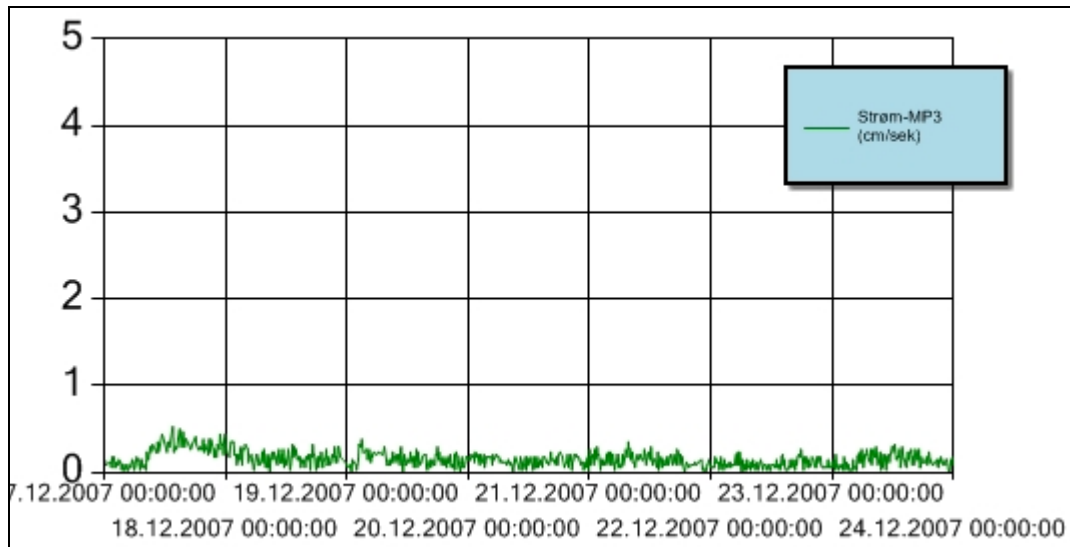
Figur 13 Strømhastighet for perioden 17. – 23. desember 2007 ved målestasjon MP3. Y-aksen angir strømhastighet i cm/sekund. Sensoren er forankret slik at den henger fritt ca. 3 m over sjøbunnen.
