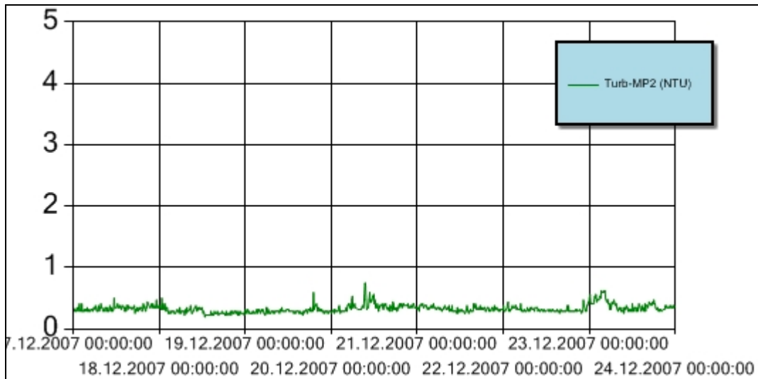
Figur 5 Turbiditet for perioden 17. – 23. desember 2007 ved målestasjon MP2. Y-aksen angir målt turbiditet (NTU). Turbiditetsensoren er plassert ca. 3 m over sjøbunnen.
