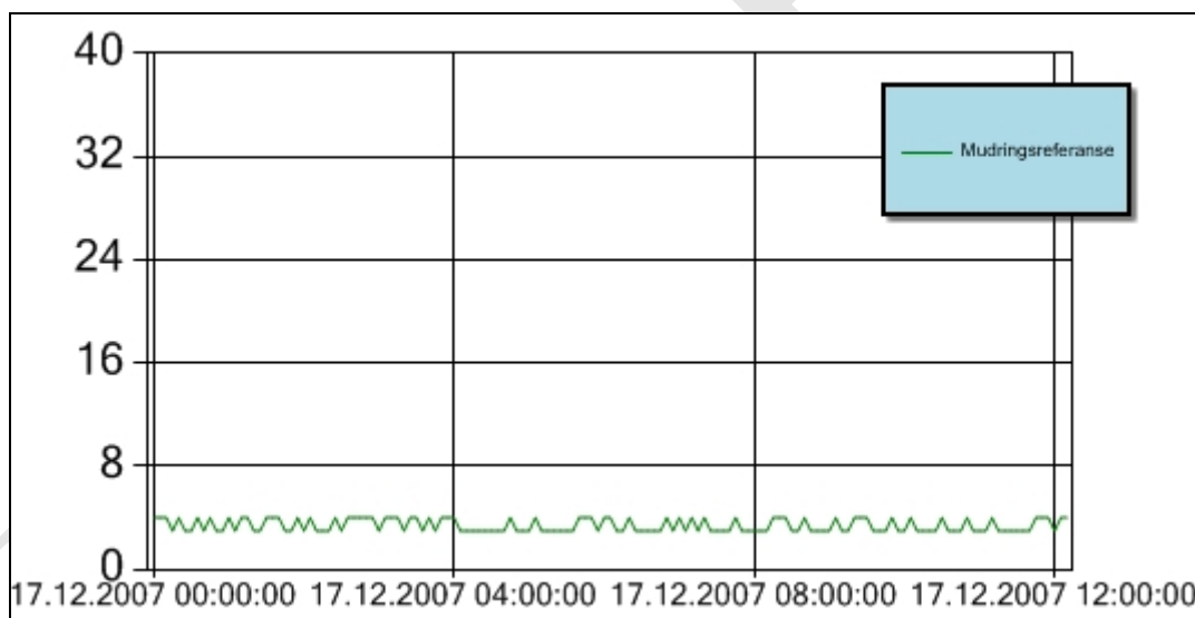
Figur 2 Turbiditet for perioden 17. – 23. desember 2007 ved referansestasjonen ved Akershusutstikkeren under mudring i Pipervika. Y-aksen angir målt turbiditet (NTU).
