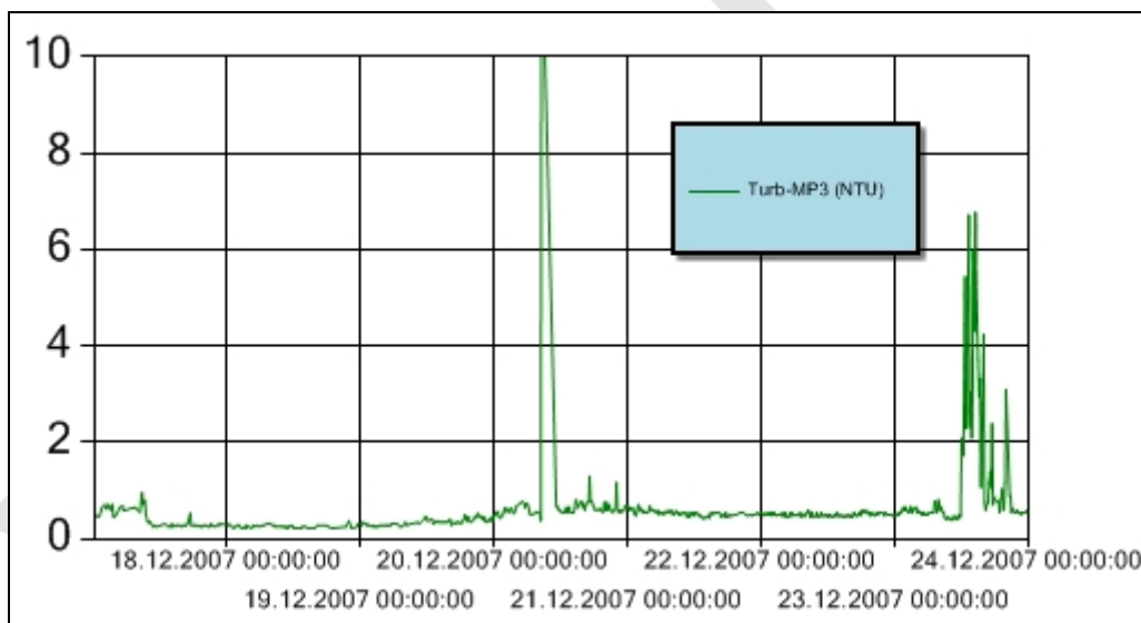
Figur 6 Turbiditet for perioden 17. – 23. desember 2007 ved målestasjon MP3. Y-aksen angir målt turbiditet (NTU). Turbiditetsensoren er plassert ca. 3 m over sjøbunnen. Merk at MP3 er oppgitt med en annen skala enn de andre målerne. Utslaget på MP3 den 20. desember skyldes forstyrrelser i forbindelse med arbeider på bøyen denne dagen.
