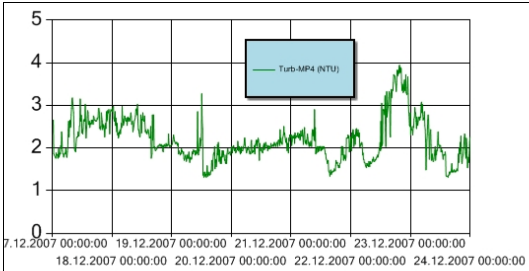
Figur 9 Turbiditet for perioden 17. – 23. desember ved målestasjon MP4. Y-aksen angir målt turbiditet (NTU). Turbiditetsensoren er plassert ca. 3 m over sjøbunnen.
