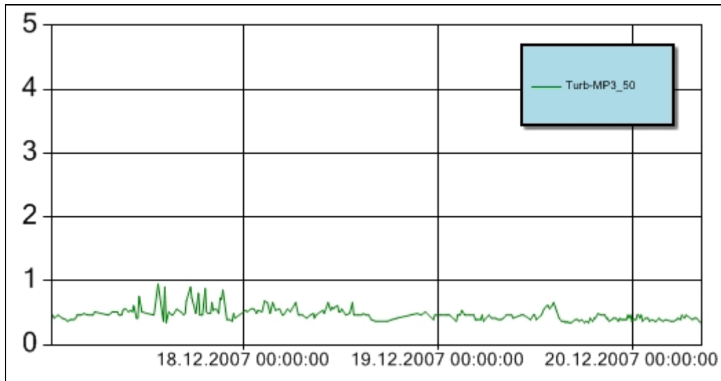
Figur 7 Turbiditet for perioden 17. – 20. desember 2007 ved målestasjon MP3_50. Y-aksen angir målt turbiditet (NTU). Turbiditetsensoren er plassert ved 50 m vanddyb.
