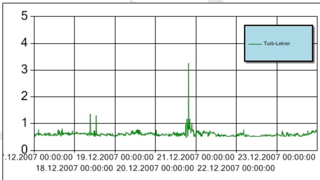
Figur 12 Turbiditet for perioden 17. – 23. desember 2007 ved H2, nedføringsenheten. Turbiditetsensoren er plassert ca. 10 m under overflata. Y-aksen angir målt turbiditet (NTU).
