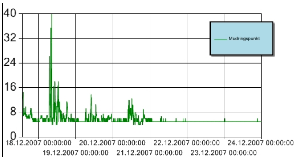
Figur 1 Turbiditet for perioden 17. – 23. desember 2007 ved mudringslekter under mudring i Pipervika. Y-aksen angir målt turbiditet (NTU). Alle stopp som følge av overskredet grenseverdi for turbiditet blir dokumentert i månedsrapport for desember.
