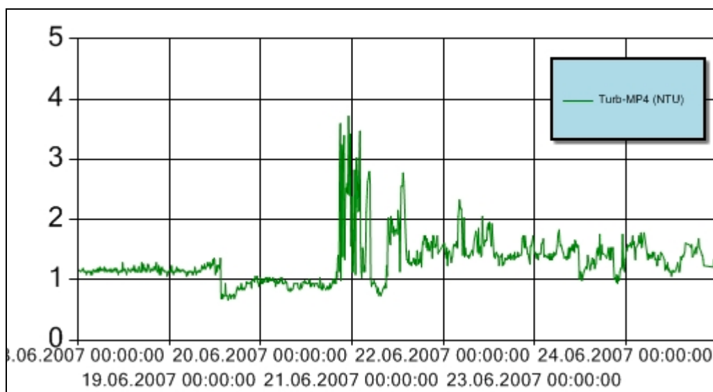
Figur 10 Turbiditet for perioden 18. – 24. juni 2007 ved målestasjon MP4. Y-aksen angir målt turbiditet (NTU). Turbiditetsensoren er plassert 3 m over sjøbunnen.
