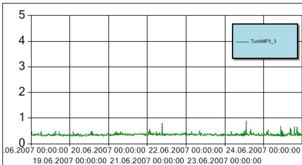
Figur 9 Turbiditet for perioden 18. – 24. juni 2007 ved målestasjon MP3_3. Y-aksen angir målt turbiditet (NTU). Turbiditetsensoren er plassert ved 40 m vanddyb.
