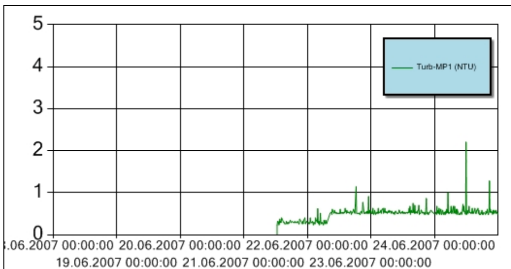
Figur 5 Turbiditet for perioden 18. – 24. juni 2007 ved målestasjon MP1. Y-aksen angir målt turbiditet (NTU). Turbiditetsensoren er plassert 3 m over sjøbunnen.
