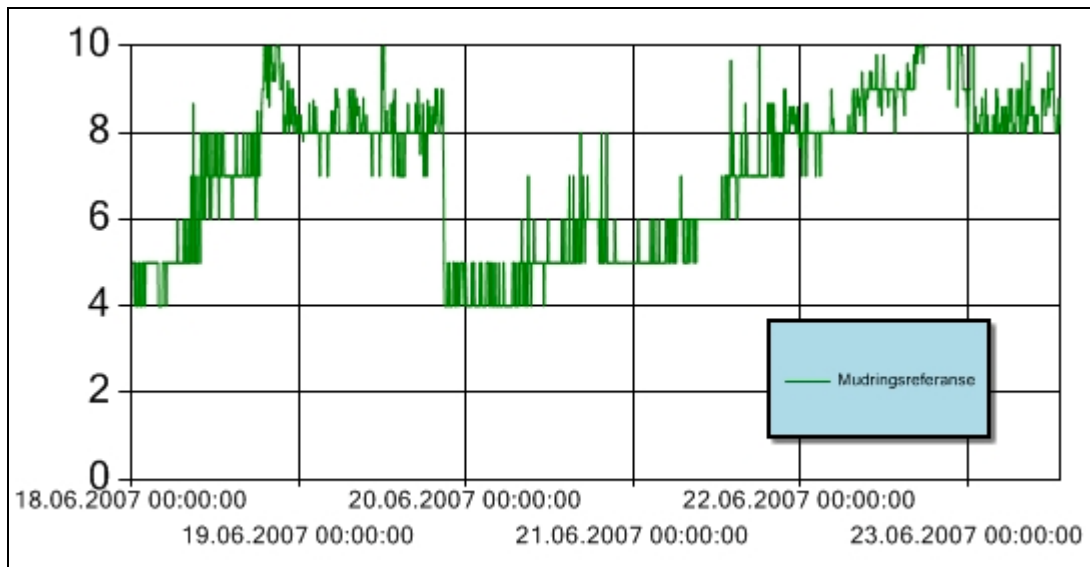
Figur 2 Turbiditet for perioden 18. - 24. juni 2007 ved referansestasjonen ved Sørengutstikkeren under mudring i Bjørvika. Y-aksen angir målt turbiditet (NTU). Høye enkeltmålinger skyldes støy.
