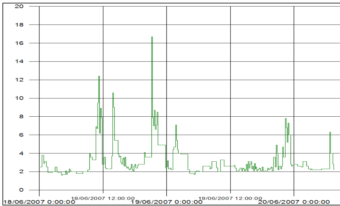
Figur 3 Turbiditet for perioden 18. - 20. juni 2007 ved mudringslekker under mudring ved Hovedøya. Y-aksen angir målt turbiditet (NTU).
