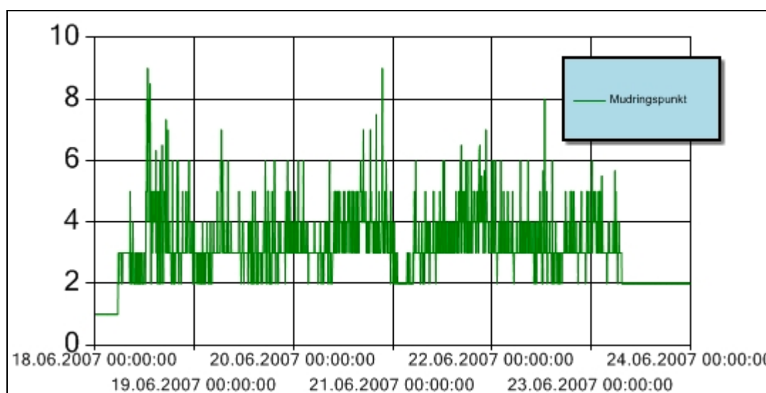
Figur 1 Turbiditet for perioden 18. - 24. juni 2007 ved mudringslekter under mudring i Bjørvika. Y-aksen angir målt turbiditet (NTU). Alle stopp som følge av overskredet grenseverdi for turbiditet blir dokumentert i månedsrapport for juni.
