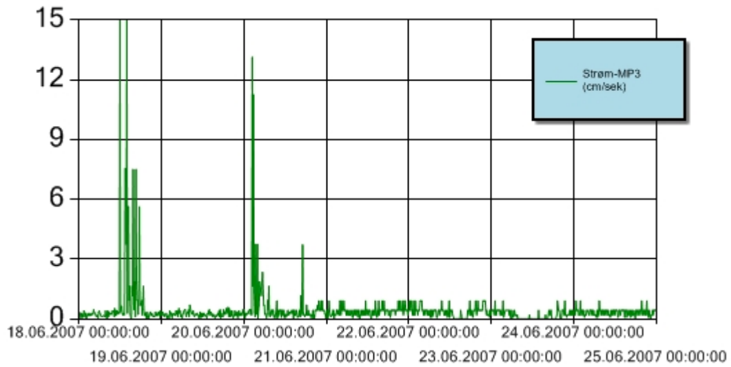
Figur 13 Strømhastighet for perioden 18. – 24. juni 2007 ved målestasjon MP3. Y-aksen angir strømhastighet i cm/sekund. Sensoren er forankret slik at den henger fritt 3 m over sjøbunnen. Høye enkeltmålinger skyldes støy.
