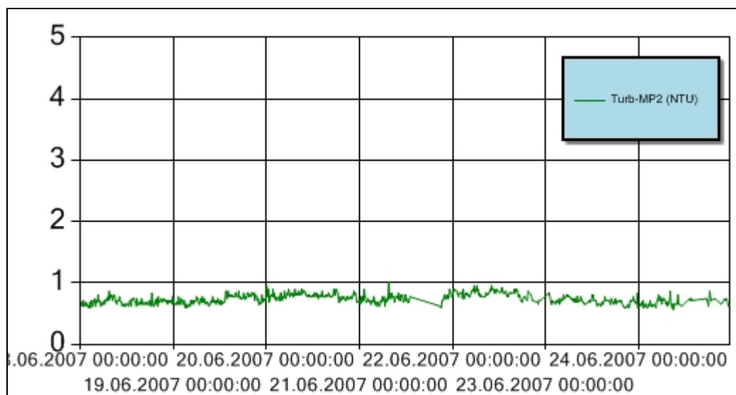
Figur 6 Turbiditet for perioden 18. – 24. juni 2007 ved målestasjon MP2. Y-aksen angir målt turbiditet (NTU). Turbiditetsensoren er plassert 3 m over sjøbunnen.
