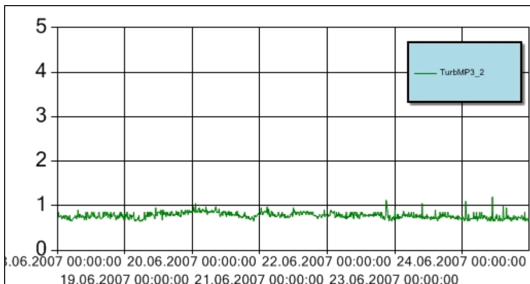
Figur 8 Turbiditet for perioden 18. – 24. juni 2007 ved målestasjon MP3_2. Y-aksen angir målt turbiditet (NTU). Turbiditetsensoren er plassert ved 50 m vanddyb.
