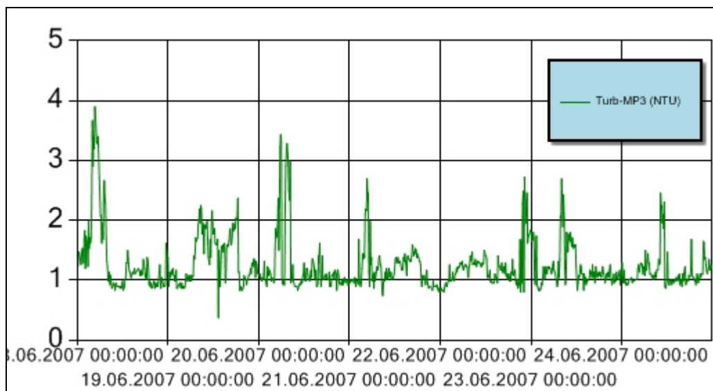
Figur 7 Turbiditet for perioden 18. – 24. juni 2007 ved målestasjon MP3. Y-aksen angir målt turbiditet (NTU). Turbiditetsensoren er plassert 3 m over sjøbunnen.
