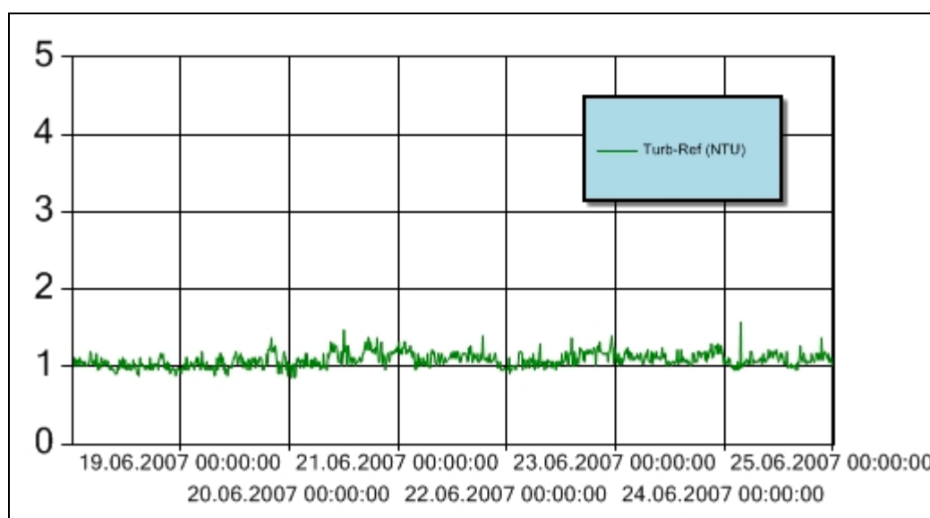
Figur 12 Turbiditet for perioden 18. – 24. juni 2007 ved referansestasjonen i Bekkelagsbassenget. Turbiditetsensoren er plassert 3 m over sjøbunnen. Y-aksen angir målt turbiditet (NTU).
