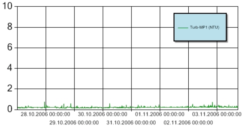
Figur 4: Turbiditet for perioden 27. oktober-3. november 2006 ved målestasjon MP1. Y-aksen angir målt turbiditet (NTU). Turbiditetsensoren er plassert 3 m over sjøbunnen. Grenseverdien for turbiditet er ikke overskredet i perioden.
