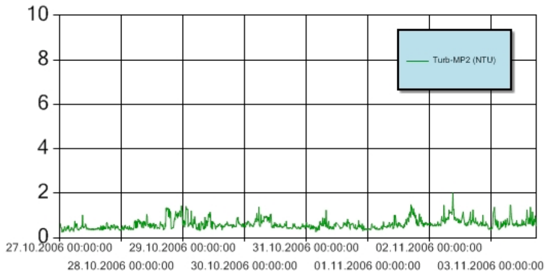
Figur 5: Turbiditet for perioden 27. oktober-3. november 2006 ved målestasjon MP2. Y-aksen angir målt turbiditet (NTU). Turbiditetsensoren er plassert 3 m over sjøbunnen. Grenseverdien for turbiditet er ikke overskredet i perioden.
