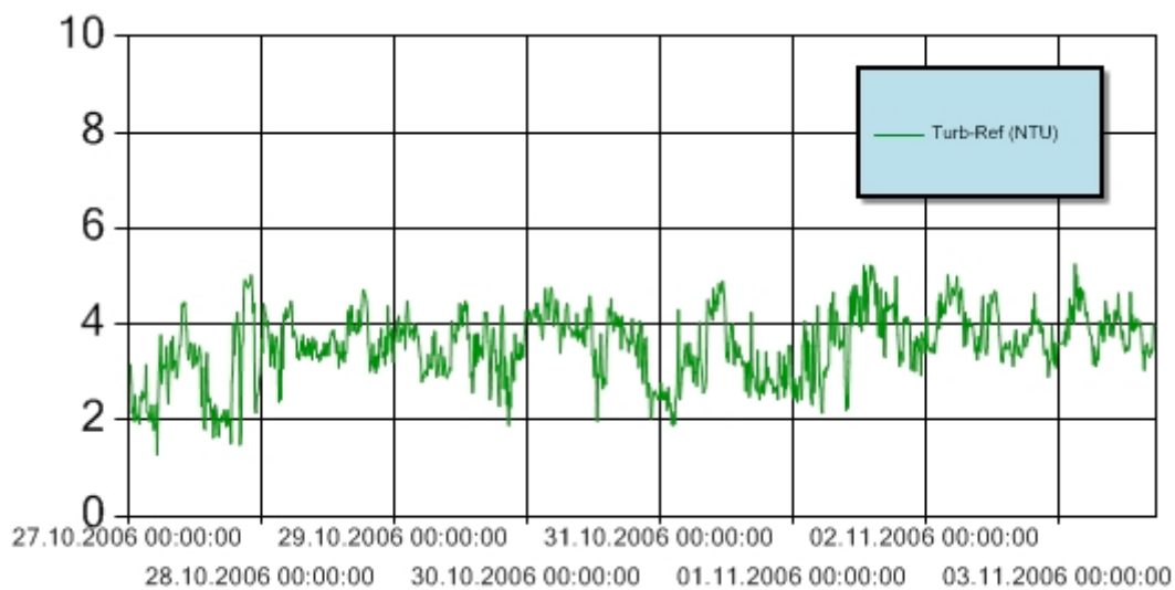
Figur 8: Turbiditet for perioden 27. oktober-3. november 2006 ved referansestasjonen i Bekkelagsbassenget. Turbiditetsensoren er plassert 3 m over sjøbunnen. Y-aksen angir målt turbiditet (NTU).
