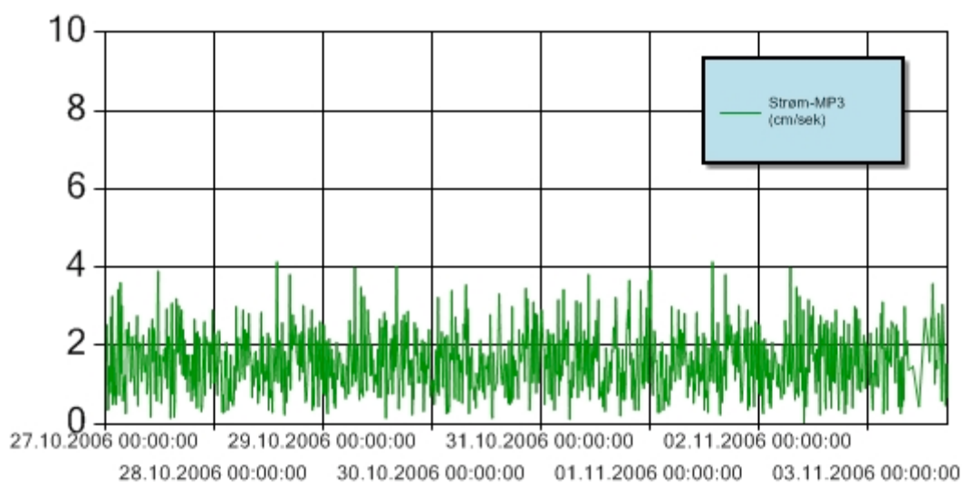
Figur 9: Strømhastighet for perioden 27. oktober-3. november 2006 ved målestasjon MP3. Y-aksen angir strømhastighet i cm/sekund. Sensoren er forankret slik at den henger fritt 3 m over sjøbunnen. Grenseverdien for strømhastighet er ikke overskredet i perioden.
