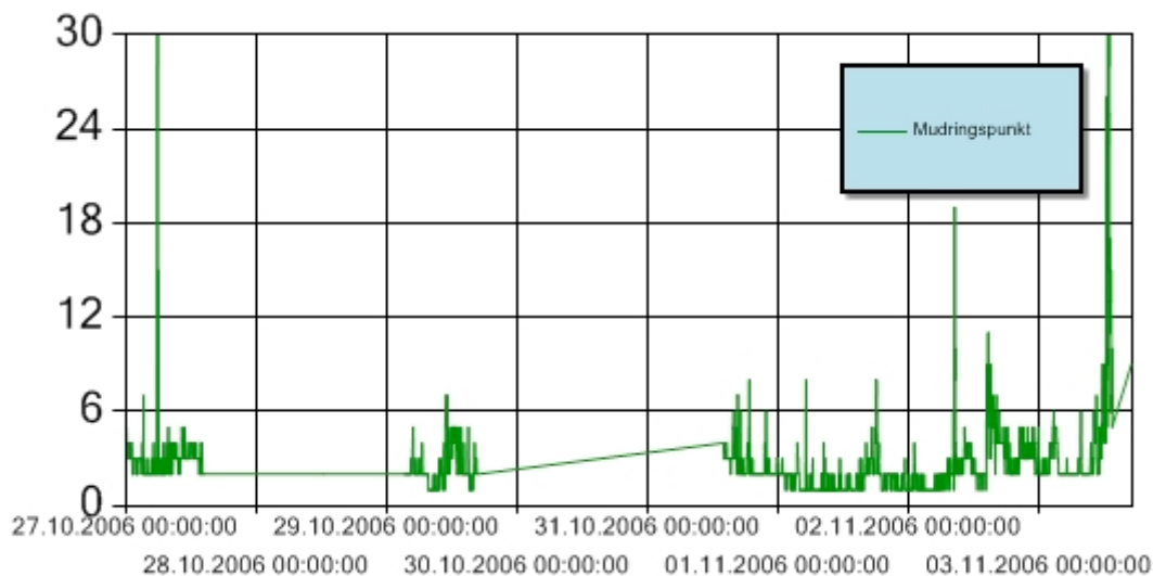
Figur 1: Turbiditet for perioden 27. oktober-3. november 2006 ved mudringslekter. Y-aksen angir målt turbiditet (NTU). Turbiditetssensoren er plassert 3 m over sjøbunnen. Alle stopp som følge av overskredet grenseverdi for turbiditet blir dokumentert i månedsrapport for september. Det blir ikke gjort registreringer av turbiditet når mudringsfartøyet ikke er i produksjon.
