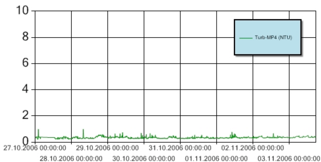
Figur 7: Turbiditet for perioden 27. oktober-3. november 2006 ved målestasjon MP4. Y-aksen angir målt turbiditet (NTU). Turbiditetsensoren er plassert 3 m over sjøbunnen. Grenseverdien for turbiditet er ikke overskredet i perioden.
