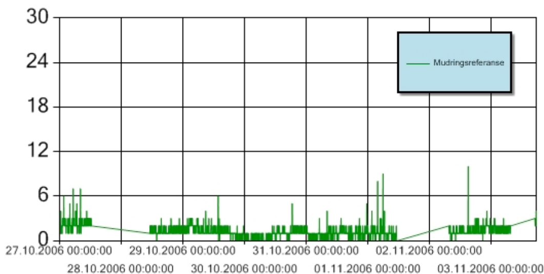
Figur 2: Turbiditet for perioden 27. oktober-3. november 2006 ved Sørengutstikkeren (referanse). Y-aksen angir målt turbiditet (NTU). Turbiditetssensoren er plassert 3 m over sjøbunnen. Ved evt. nedetid i referansemålingene blir bakgrunnsverdien antatt lik 1 NTU ved vurdering av overskridelser av grenseverdi for turbiditet.
