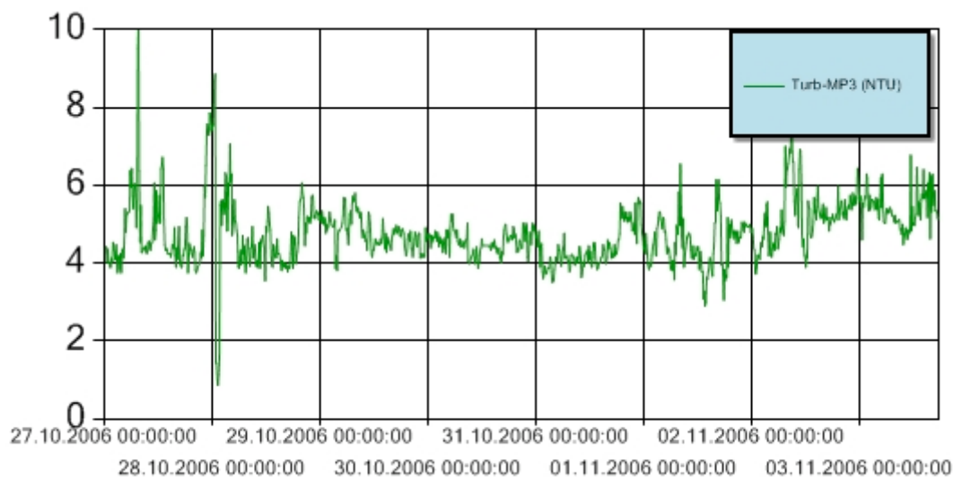
Figur 6: Turbiditet for perioden 27. oktober-3. november 2006 ved målestasjon MP3. Y-aksen angir målt turbiditet (NTU). Turbiditetsensoren er plassert 3 m over sjøbunnen. Grenseverdien for turbiditet er ikke overskredet i perioden. Det naturlige bakgrunnsnivået i bunnvannet i området er naturlig forhøyet (se bakgrunnsdata i figur 8) som følge av at oksygenkonsentrasjonen i vannmassene dypere enn ca 60 m er tilnærmet lik null.
