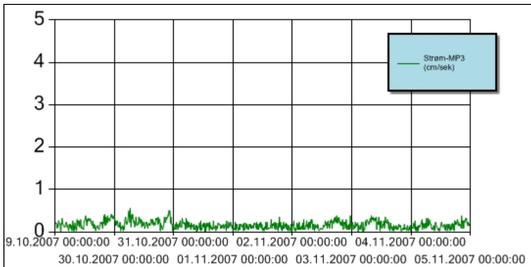
Figur 14 Strømhastighet for perioden 29. oktober – 4. november 2007 ved målestasjon MP3. Y-aksen angir strømhastighet i cm/sekund. Sensoren er forankret slik at den henger fritt ca. 3 m over sjøbunnen.
