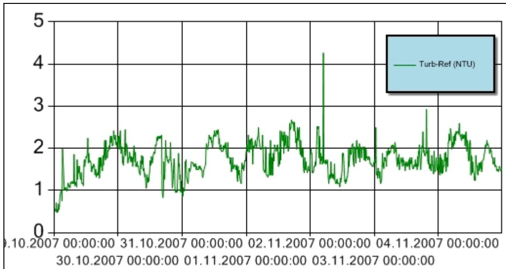
Figur 13 Turbiditet for perioden 29. oktober – 4. november 2007 ved referansestasjonen i Bekkelagsbassenget. Turbiditetsensoren er plassert ca. 3 m over sjøbunnen. Y-aksen angir målt turbiditet (NTU). Høye enkeltverdier skyldes støy.
