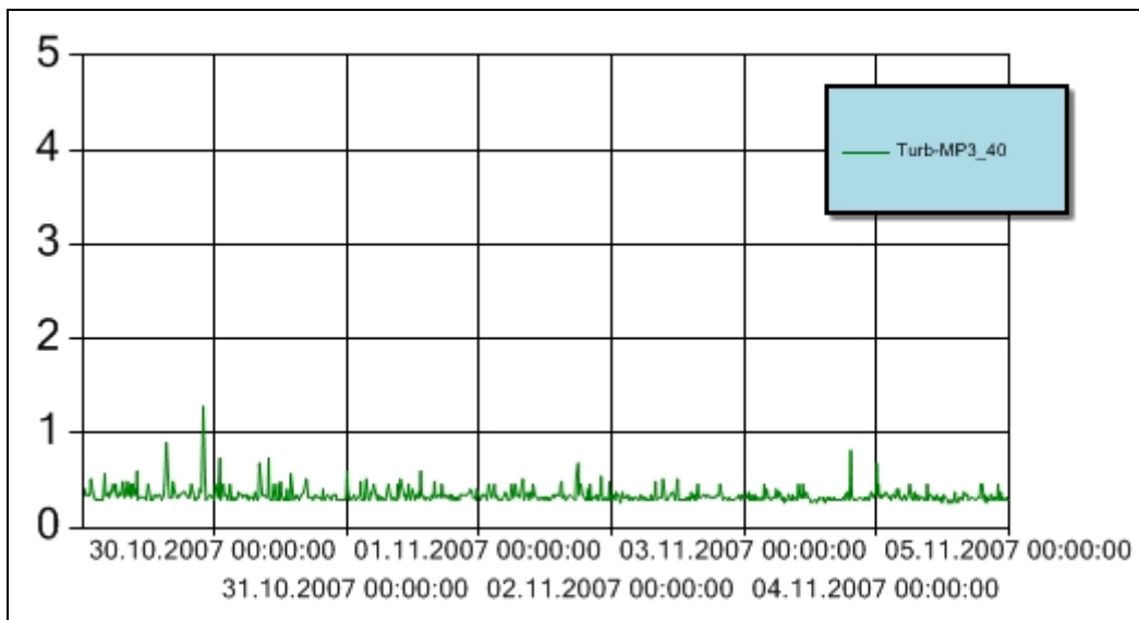
Figur 10 Turbiditet for perioden 29. oktober – 4. november 2007 ved målestasjon MP3_40. Y-aksen angir målt turbiditet (NTU). Turbiditetsensoren er plassert ved 40 m vannndyp.
