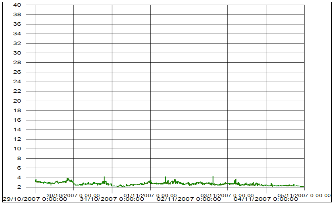
Figur 4 Turbiditet for perioden 29. oktober – 4. november 2007 ved referansestasjonen ved serviceflåten i Bestumkilen under mudring i Bestumkilen. Y-aksen angir målt turbiditet (NTU).
