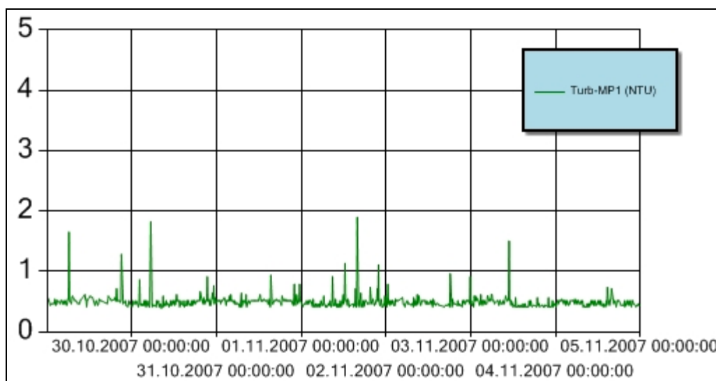
Figur 6 Turbiditet for perioden 29. oktober – 4. november 2007 ved målestasjon MP1. Y-aksen angir målt turbiditet (NTU). Turbiditetsensoren er plassert ca. 3 m over sjøbunnen.
