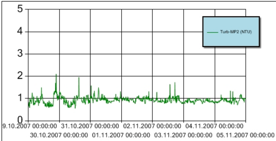
Figur 7 Turbiditet for perioden 29. oktober – 4. november 2007 ved målestasjon MP2. Y-aksen angir målt turbiditet (NTU). Turbiditetsensoren er plassert ca. 3 m over sjøbunnen.
