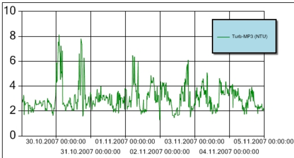
Figur 8 Turbiditet for perioden 29. oktober – 4. november 2007 ved målestasjon MP3. Y-aksen angir målt turbiditet (NTU). Turbiditetsensoren er plassert ca. 3 m over sjøbunnen. Merk at MP3 er oppgitt med en annen skala enn de andre målerne.
