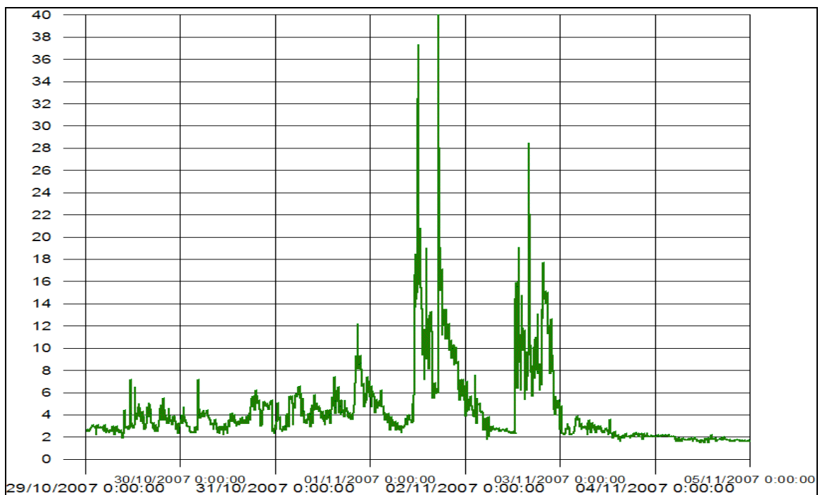
Figur 3 Turbiditet for perioden 29. oktober – 4. november 2007 ved mudringslekter i Bestumkilen. Y-aksen angir målt turbiditet (NTU). Alle stopp som følge av overskredet grenseverdi for turbiditet blir dokumentert i månedsrapport for november.
