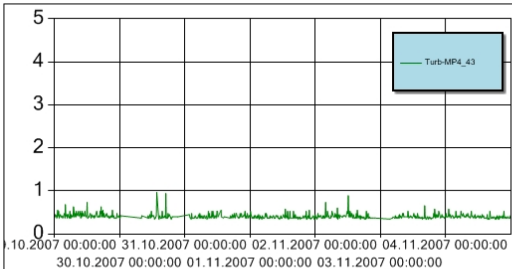
Figur 12 Turbiditet for perioden 29. oktober – 4. november 2007 ved målestasjon MP4_43. Y-aksen angir målt turbiditet (NTU). Turbiditetsensoren er plassert ved 43 m vann dybde.
