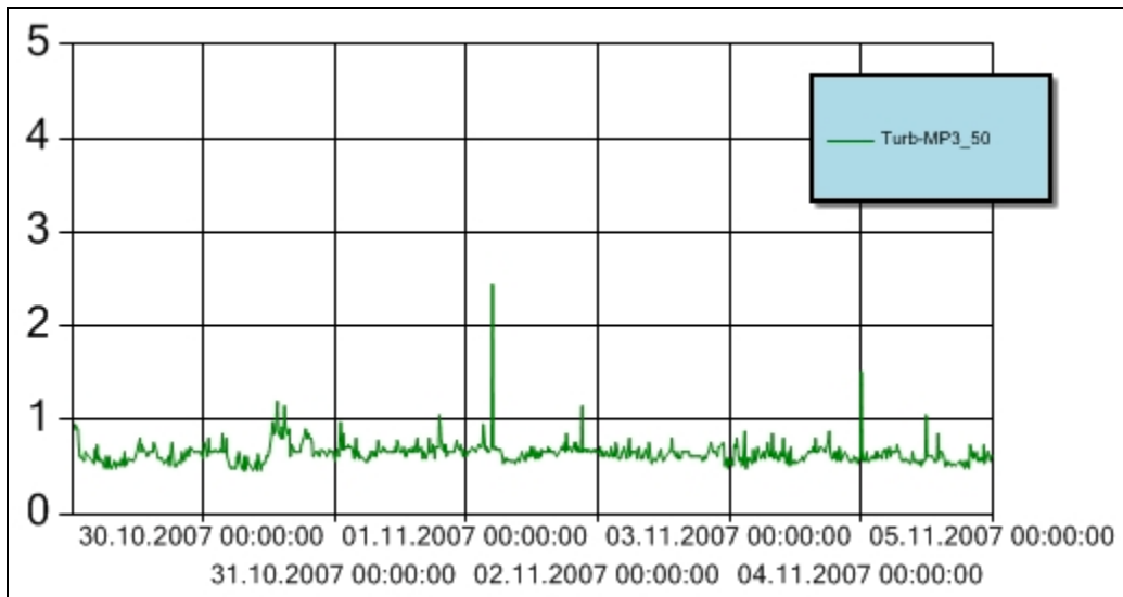
Figur 9 Turbiditet for perioden 29. oktober – 4. november 2007 ved målestasjon MP3_50. Y-aksen angir målt turbiditet (NTU). Turbiditetsensoren er plassert ved 50 m vannndyp. Høye enkeltmålinger skyldes støy.
