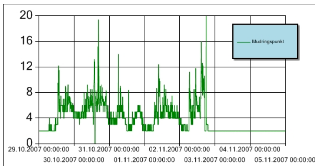
Figur 1 Turbiditet for perioden 29. oktober – 4. november 2007 ved mudringslekter under mudring i Lohavn. Y-aksen angir målt turbiditet (NTU). Alle stopp som følge av overskredet grenseverdi for turbiditet blir dokumentert i månedsrapport for november.
