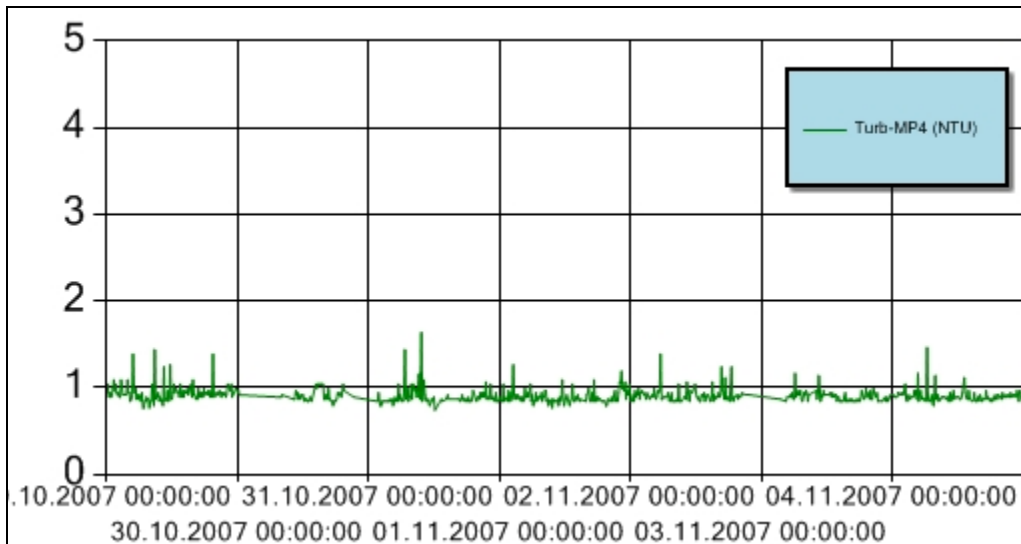
Figur 11 Turbiditet for perioden 29. oktober – 4. november ved målestasjon MP4. Y-aksen angir målt turbiditet (NTU). Turbiditetsensoren er plassert ca. 3 m over sjøbunnen.
