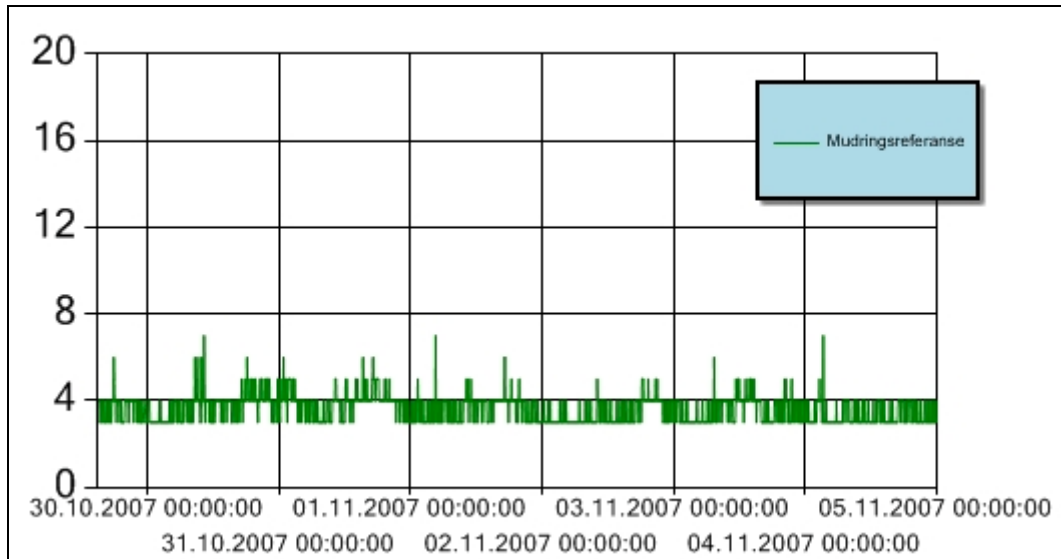
Figur 2 Turbiditet for perioden 29. oktober – 4. november 2007 ved referansestasjonen ved Sørengutstikkeren under mudring i Lohavn. Y-aksen angir målt turbiditet (NTU).
