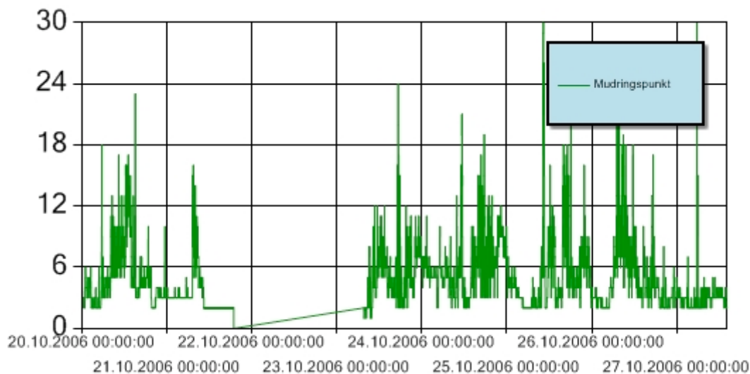
Figur 1: Turbiditet for perioden 20.-27 oktober 2006 ved mudringslekter. Y-aksen angir målt turbiditet (NTU). Turbiditetssensoren er plassert 3 m over sjøbunnen. Alle stopp som følge av overskredet grenseverdi for turbiditet blir dokumentert i månedsrapport for september. Det blir ikke gjort registreringer av turbiditet når mudringsfartøyet ikke er i produksjon.
