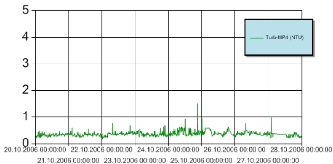
Figur 7: Turbiditet for perioden 20.-27 oktober 2006 ved målestasjon MP4. Y-aksen angir målt turbiditet (NTU). Turbiditetsensoren er plassert 3 m over sjøbunnen. Grenseverdien for turbiditet er ikke overskredet i perioden.
