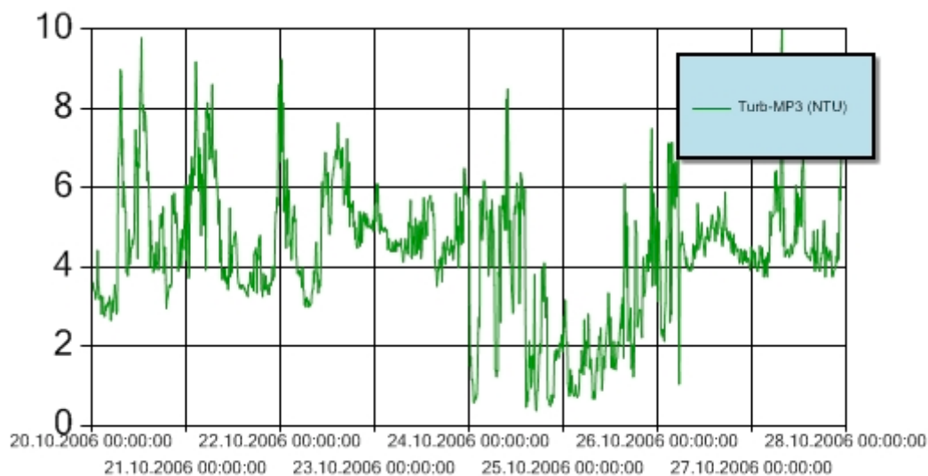
Figur 6: Turbiditet for perioden 20.-27 oktober 2006 ved målestasjon MP3. Y-aksen angir målt turbiditet (NTU). Turbiditetsensoren er plassert 3 m over sjøbunnen. Grenseverdien for turbiditet er ikke overskredet i perioden.
