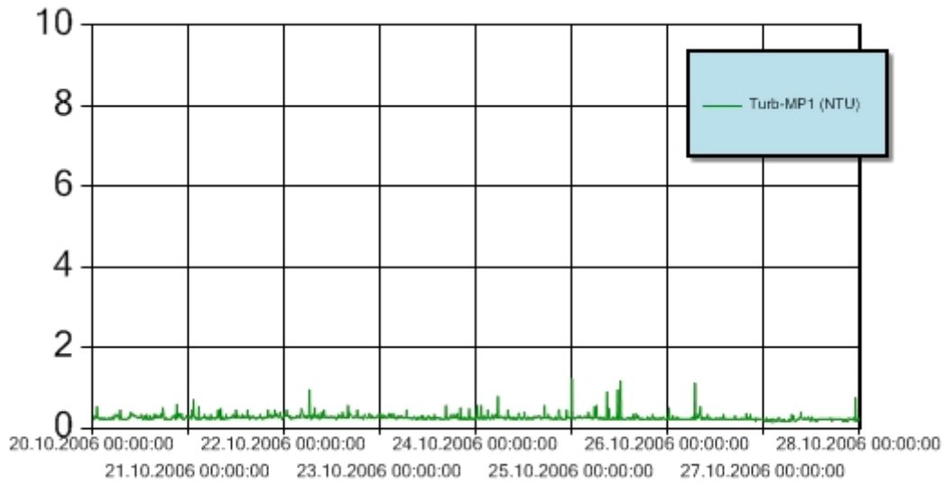
Figur 4: Turbiditet for perioden 20.-27 oktober 2006 ved målestasjon MP1. Y-aksen angir målt turbiditet (NTU). Turbiditetsensoren er plassert 3 m over sjøbunnen. Grenseverdien for turbiditet er ikke overskredet i perioden.
