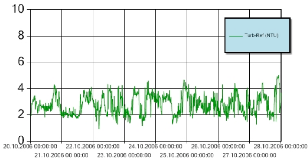
Figur 8: Turbiditet for perioden 20.-27 oktober 2006 ved referansestasjonen i Bekkelagsbassenget. Turbiditetsensoren er plassert 3 m over sjøbunnen. Y-aksen angir målt turbiditet (NTU).
