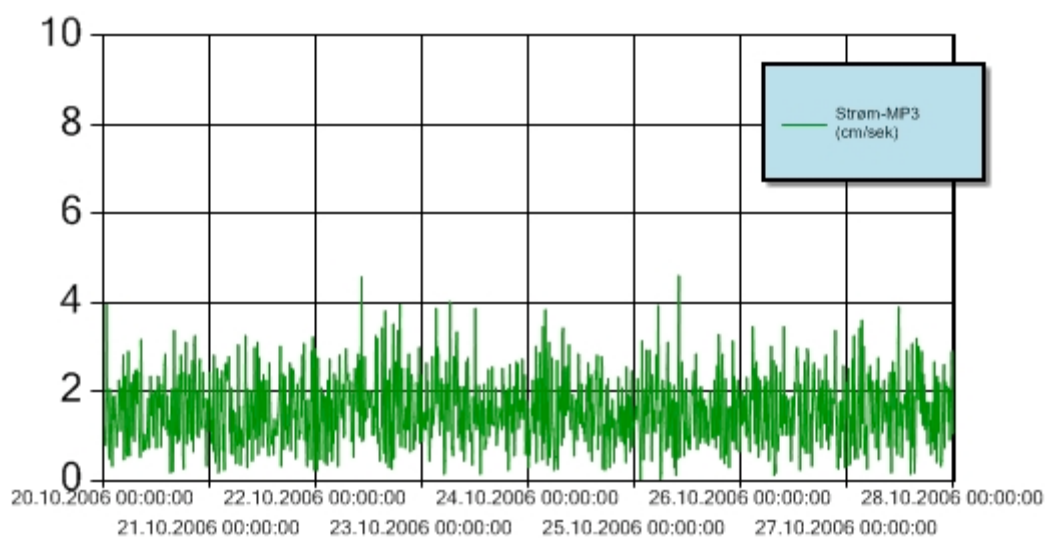
Figur 9: Strømhastighet for perioden 20.-27 oktober 2006 ved målestasjon MP3. Y-aksen angir strømhastighet i cm/sekund. Sensoren er forankret slik at den henger fritt 3 m over sjøbunnen. Grenseverdien for strømhastighet er ikke overskredet i perioden.
