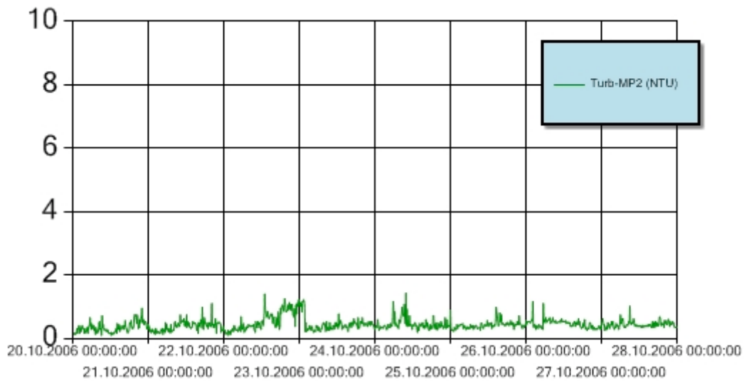
Figur 5: Turbiditet for perioden 20.-27 oktober 2006 ved målestasjon MP2. Y-aksen angir målt turbiditet (NTU). Turbiditetsensoren er plassert 3 m over sjøbunnen. Grenseverdien for turbiditet er ikke overskredet i perioden.
