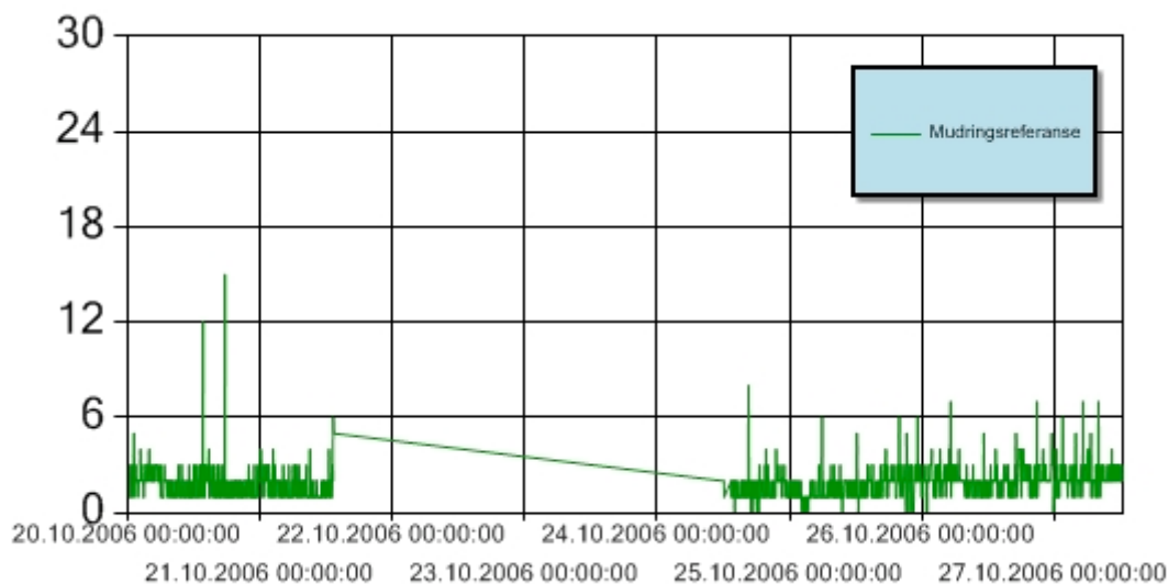
Figur 2: Turbiditet for perioden 20.-27 oktober 2006 ved Sørengutstikkeren (referanse). Y-aksen angir målt turbiditet (NTU). Turbiditetssensoren er plassert 3 m over sjøbunnen. Ved evt. nedetid i referansemålingene blir bakgrunnsverdien antatt lik 1 NTU ved vurdering av overskridelser av grenseverdi for turbiditet.
