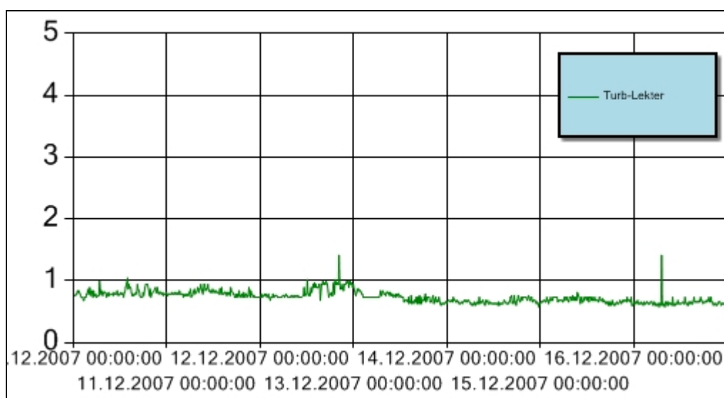
Figur 12 Turbiditet for perioden 10. – 16. desember 2007 ved H2, nedføringsenheten. Turbiditetsensoren er plassert ca. 10 m under overflata. Y-aksen angir målt turbiditet (NTU).
