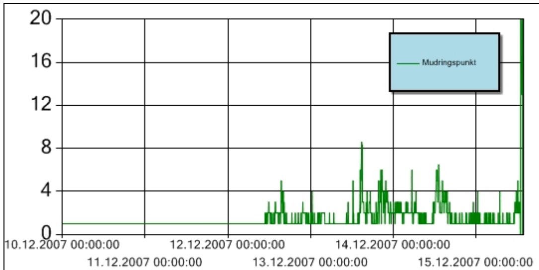
Figur 1 Turbiditet for perioden 10. – 16. desember 2007 ved mudringsleker under mudring i Pipervika. Y-aksen angir målt turbiditet (NTU). Alle stopp som følge av overskredet grenseverdi for turbiditet blir dokumentert i månedsrapport for desember.
