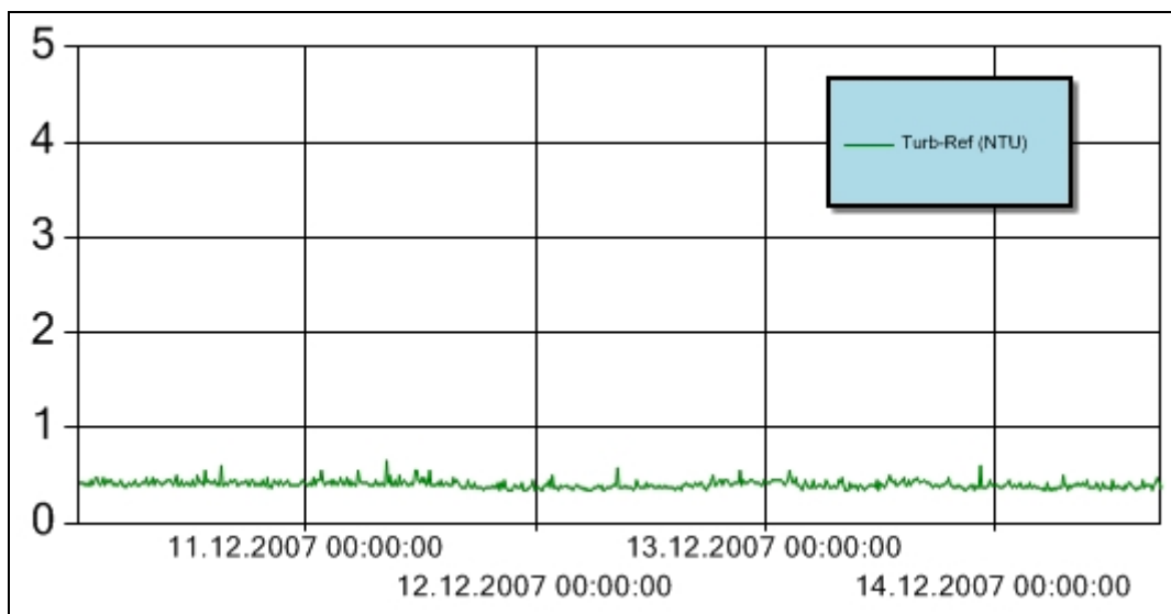
Figur 11 Turbiditet for perioden 10. – 15. desember 2007 ved referansestasjonen i Bekkelagsbassenget. Turbiditetsensoren er plassert ca. 3 m over sjøbunnen. Y-aksen angir målt turbiditet (NTU). Måleren sluttet å fungere den 15. desember.
