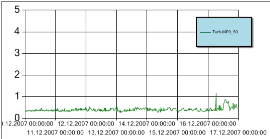
Figur 7 Turbiditet for perioden 10. – 16. desember 2007 ved målestasjon MP3_50. Y-aksen angir målt turbiditet (NTU). Turbiditetsensoren er plassert ved 50 m vanddyb. Høye enkeltmålinger skyldes støy.
