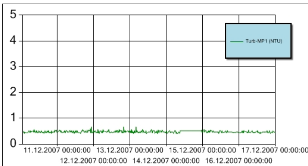
Figur 4 Turbiditet for perioden 10. – 16. desember 2007 ved målestasjon MP1. Y-aksen angir målt turbiditet (NTU). Turbiditetsensoren er plassert ca. 3 m over sjøbunnen.
