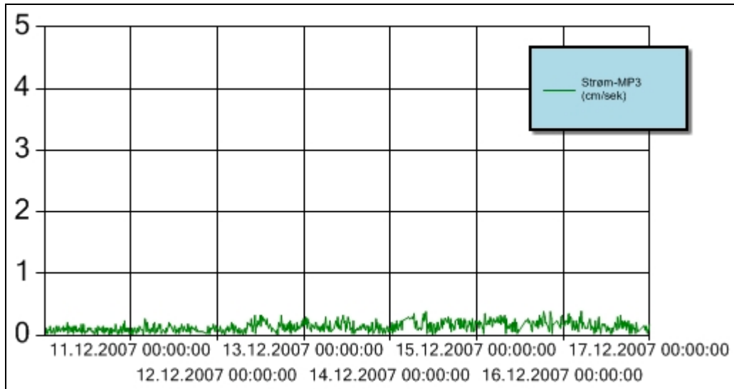
Figur 13 Strømhastighet for perioden 10. – 16. desember 2007 ved målestasjon MP3. Y-aksen angir strømhastighet i cm/sekund. Sensoren er forankret slik at den henger fritt ca. 3 m over sjøbunnen.
