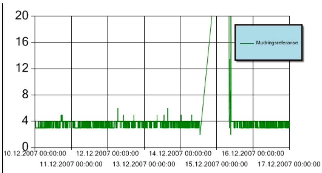
Figur 2 Turbiditet for perioden 10. – 16. desember 2007 ved referansestasjonen ved Akershusutstikkeren under mudring i Pipervika. Y-aksen angir målt turbiditet (NTU).
