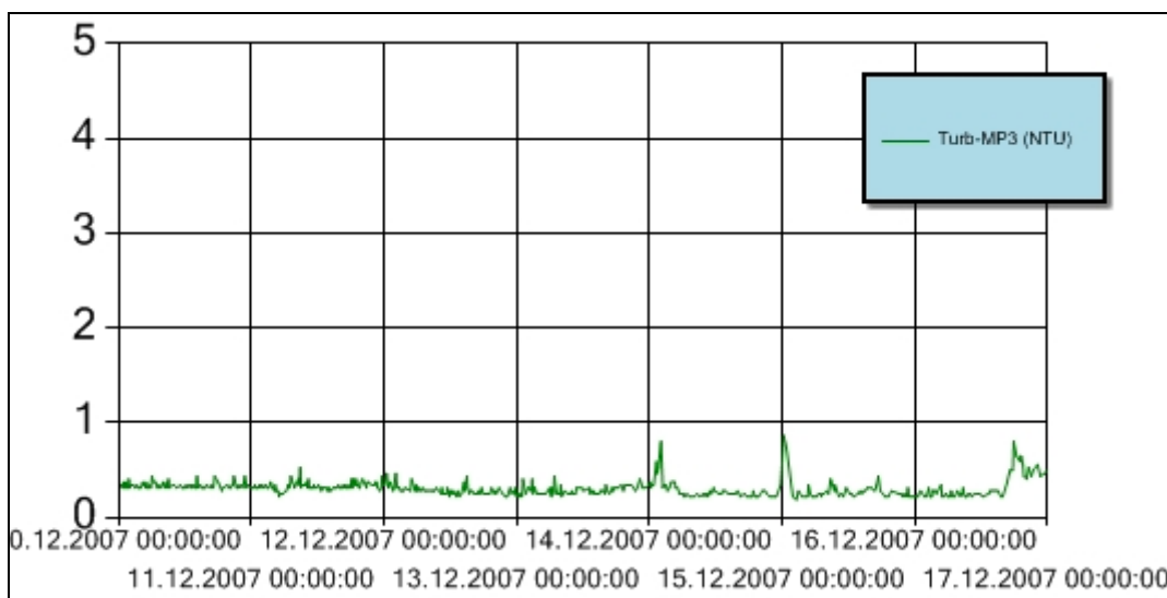
Figur 6 Turbiditet for perioden 10. – 16. desember 2007 ved målestasjon MP3. Y-aksen angir målt turbiditet (NTU). Turbiditetsensoren er plassert ca. 3 m over sjøbunnen.
