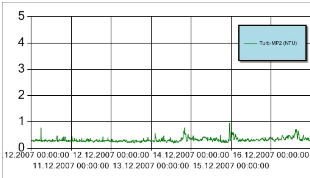
Figur 5 Turbiditet for perioden 10. – 16. desember 2007 ved målestasjon MP2. Y-aksen angir målt turbiditet (NTU). Turbiditetsensoren er plassert ca. 3 m over sjøbunnen.
