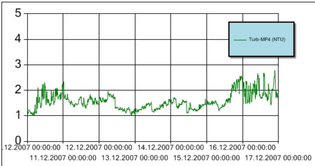
Figur 9 Turbiditet for perioden 10. – 16. desember ved målestasjon MP4. Y-aksen angir målt turbiditet (NTU). Turbiditetsensoren er plassert ca. 3 m over sjøbunnen.
