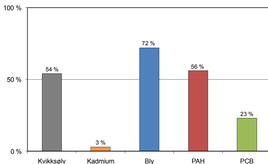
Figur 6 Forbruk av miljøbudsjettet for dypvannsdeponiet basert på miljøregnskap februar 2006 til oktober 2008 (NGI rapport 20051785-55).
