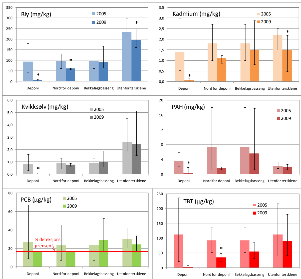
Figur 1 Sedimentkonsentrasjoner før og etter etablering av dypvannsdeponiet i og utenfor Bekkelagsbassenget (se vedlegg A). Figuren viser gjennomsnittskonsentrasjonen samt høyest og lavest verdi (* statistisk signifikant endring).
