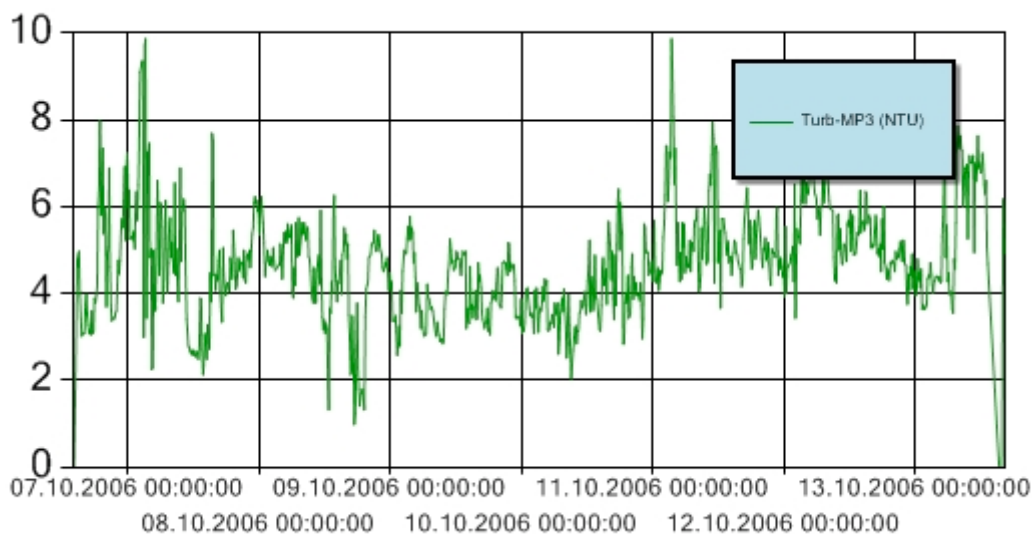
Figur 6: Turbiditet for perioden 6.-13. oktober 2006 ved målestasjon MP3. Y-aksen angir målt turbiditet (NTU). Turbiditetsensoren er plassert 3 m over sjøbunnen. Arbeidene ble stanset 13/10-06 pga. høy turbiditet.
