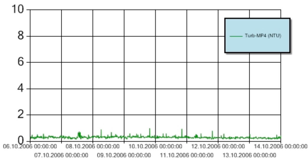
Figur 7: Turbiditet for perioden 6.-13. oktober 2006 ved målestasjon MP4. Y-aksen angir målt turbiditet (NTU). Turbiditetsensoren er plassert 3 m over sjøbunnen. Grenseverdien for turbiditet er ikke overskredet i perioden.
