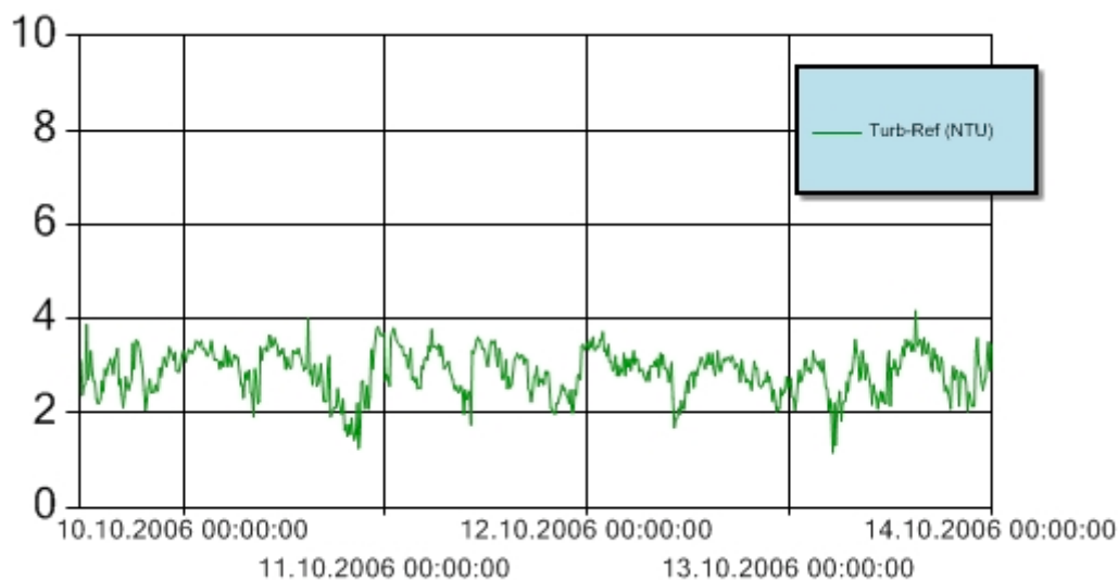
Figur 8: Turbiditet for perioden 6.-13. oktober 2006 ved referansestasjonen. Turbiditetsensoren er plassert 3 m over sjøbunnen. Y-aksen angir målt turbiditet (NTU).
