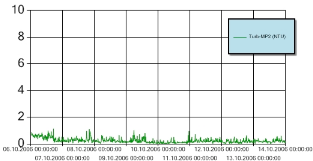
Figur 5: Turbiditet for perioden 6.-13. oktober 2006 ved målestasjon MP2. Y-aksen angir målt turbiditet (NTU). Turbiditetsensoren er plassert 3 m over sjøbunnen. Grenseverdien for turbiditet er ikke overskredet i perioden.
