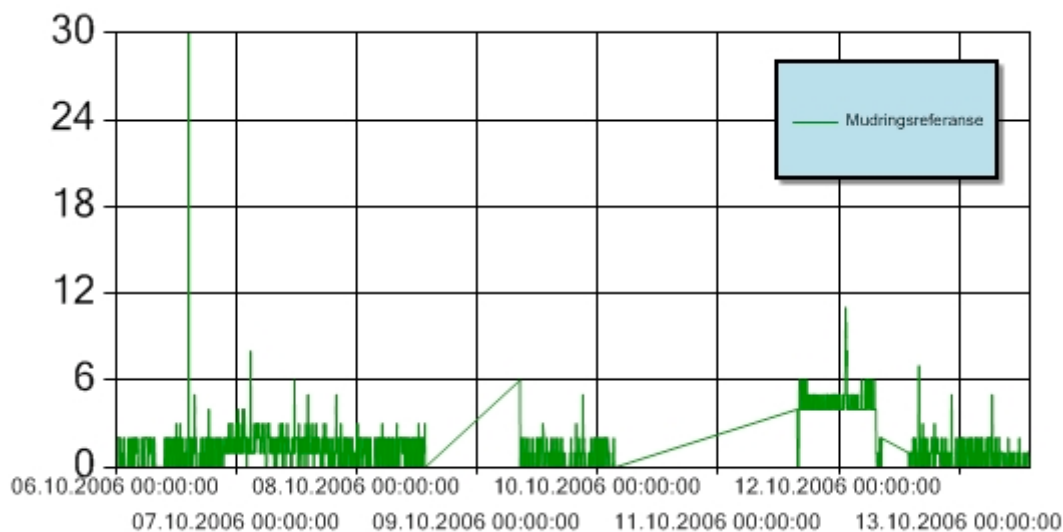
Figur 2: Turbiditet for perioden 6.-13. oktober 2006 ved Sørengutstikkeren (referanse). Y-aksen angir målt turbiditet (NTU). Turbiditetssensoren er plassert 3 m over sjøbunnen.
