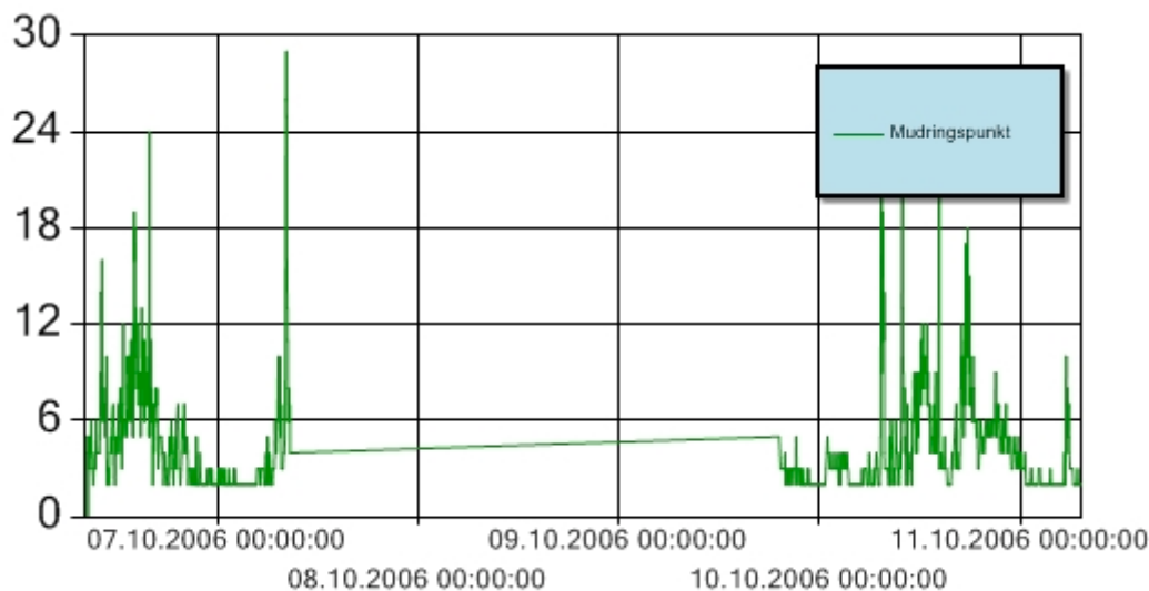
Figur 1: Turbiditet for perioden 6.-13. oktober 2006 ved mudringslekter. Y-aksen angir målt turbiditet (NTU). Turbiditetssensoren er plassert 3 m over sjøbunnen. Alle stopp som følge av overskredet grenseverdi for turbiditet blir dokumentert i månedsrapport for september. Det blir ikke gjort registreringer av turbiditet når mudringsfartøyet ikke er i produksjon.
