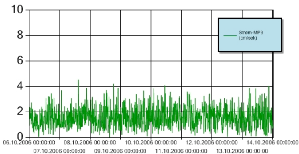
Figur 9: Strømhastighet for perioden 6.-13. oktober 2006 ved målestasjon MP3. Y-aksen angir strømhastighet i cm/sekund. Sensoren er forankret slik at den henger fritt 3 m over sjøbunnen. Grenseverdien for strømhastighet er ikke overskredet i perioden.
