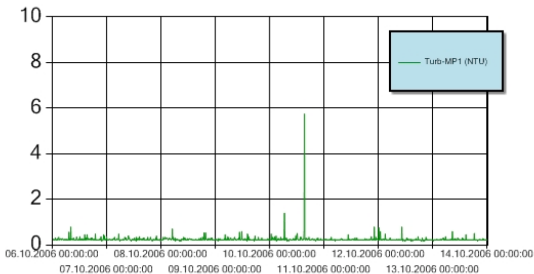
Figur 4: Turbiditet for perioden 6.-13. oktober 2006 ved målestasjon MP1. Y-aksen angir målt turbiditet (NTU). Turbiditetsensoren er plassert 3 m over sjøbunnen. Grenseverdien for turbiditet er ikke overskredet i perioden.
