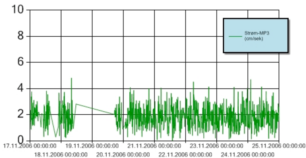
Figur 8: Strømhastighet for perioden 17.-24. november 2006 ved målestasjon MP3. Y-aksen angir strømhastighet i cm/sekund. Sensoren er forankret slik at den henger fritt 3 m over sjøbunnen. Grenseverdien for strømhastighet er ikke overskredet i perioden. Det har i perioden vært noe nedetid på instrumentet.
