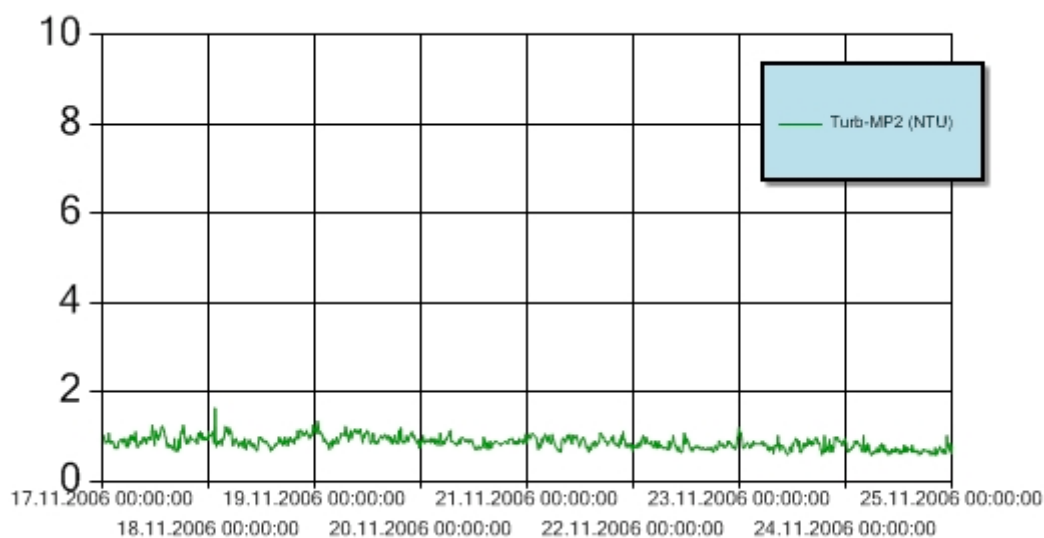
Figur 4: Turbiditet for perioden 17.-24. november 2006 ved målestasjon MP2. Y-aksen angir målt turbiditet (NTU). Turbiditetsensoren er plassert 3 m over sjøbunnen. Grenseverdien for turbiditet er ikke overskredet i perioden.
