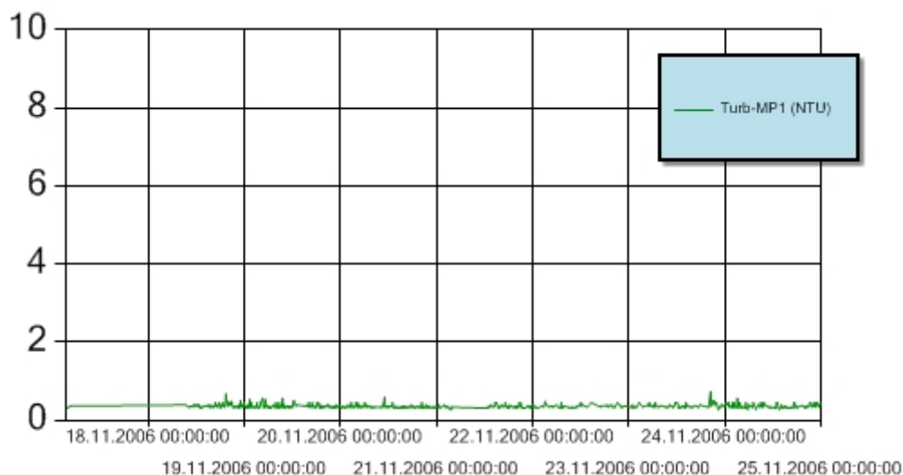
Figur 3: Turbiditet for perioden 17.-24. november 2006 ved målestasjon MP1. Y-aksen angir målt turbiditet (NTU). Turbiditetsensoren er plassert 3 m over sjøbunnen. Grenseverdien for turbiditet er ikke overskredet i perioden.
