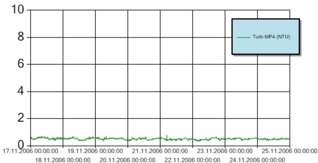
Figur 6: Turbiditet for perioden 17.-24. november 2006 ved målestasjon MP4. Y-aksen angir målt turbiditet (NTU). Turbiditetsensoren er plassert 3 m over sjøbunnen. Grenseverdien for turbiditet er ikke overskredet i perioden.
