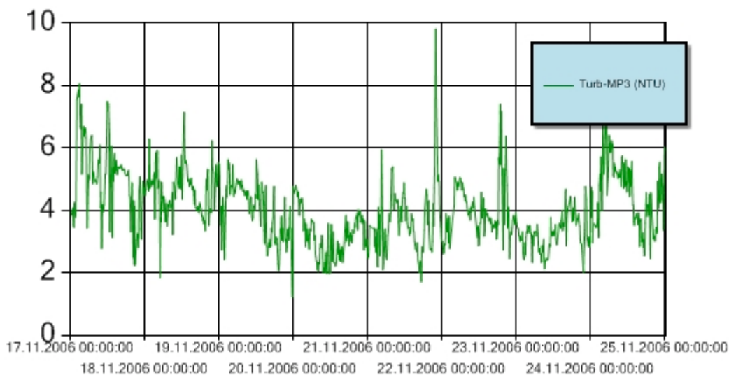
Figur 5: Turbiditet for perioden 17.-24. november 2006 ved målestasjon MP3. Y-aksen angir målt turbiditet (NTU). Turbiditetsensoren er plassert 3 m over sjøbunnen. Det naturlige bakgrunnsnivået i bunnvannet i området er naturlig forhøyet (se bakgrunnsdata i figur 8) som følge av at oksygenkonsentrasjonen i vannmassene dypere enn ca 60 m er tilnærmet lik null.
