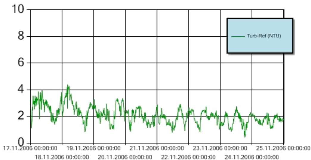
Figur 7: Turbiditet for perioden 17.-24. november 2006 ved referansestasjonen i Bekkelagsbassenget. Turbiditetsensoren er plassert 3 m over sjøbunnen. Y-aksen angir målt turbiditet (NTU). Det er naturlig høy turbiditet i bunnvannet som følge av at oksygenkonsentrasjonen er tilnærmet lik null.
