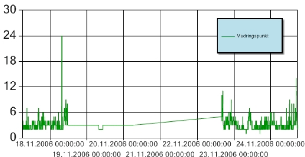
Figur 1: Turbiditet for perioden 17.-24. november 2006 ved mudringslekter. Y-aksen angir målt turbiditet (NTU). Turbiditetssensoren er plassert 3 m over sjøbunnen. Alle stopp som følge av overskredet grenseverdi for turbiditet blir dokumentert i månedsrapporten. Det blir ikke gjort registreringer av turbiditet når mudringsfartøyet ikke er i produksjon.
