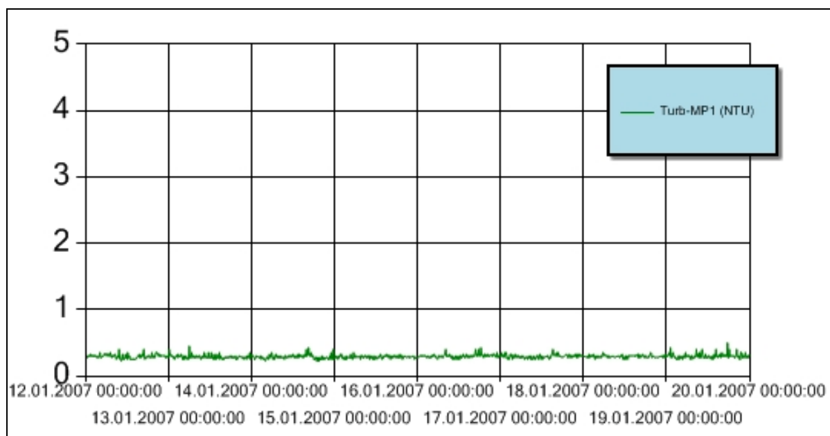
Figur 3 Turbiditet for perioden 12.-19. januar 2007 ved målestasjon MP1. Y-aksen angir målt turbiditet (NTU). Turbiditetsensoren er plassert 3 m over sjøbunnen.
