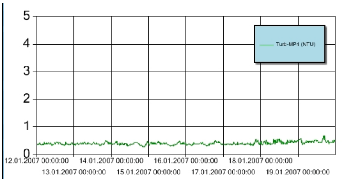
Figur 6 Turbiditet for perioden 12.-19. januar 2007 ved målestasjon MP4. Y-aksen angir målt turbiditet (NTU). Turbiditetsensoren er plassert 3 m over sjøbunnen.
