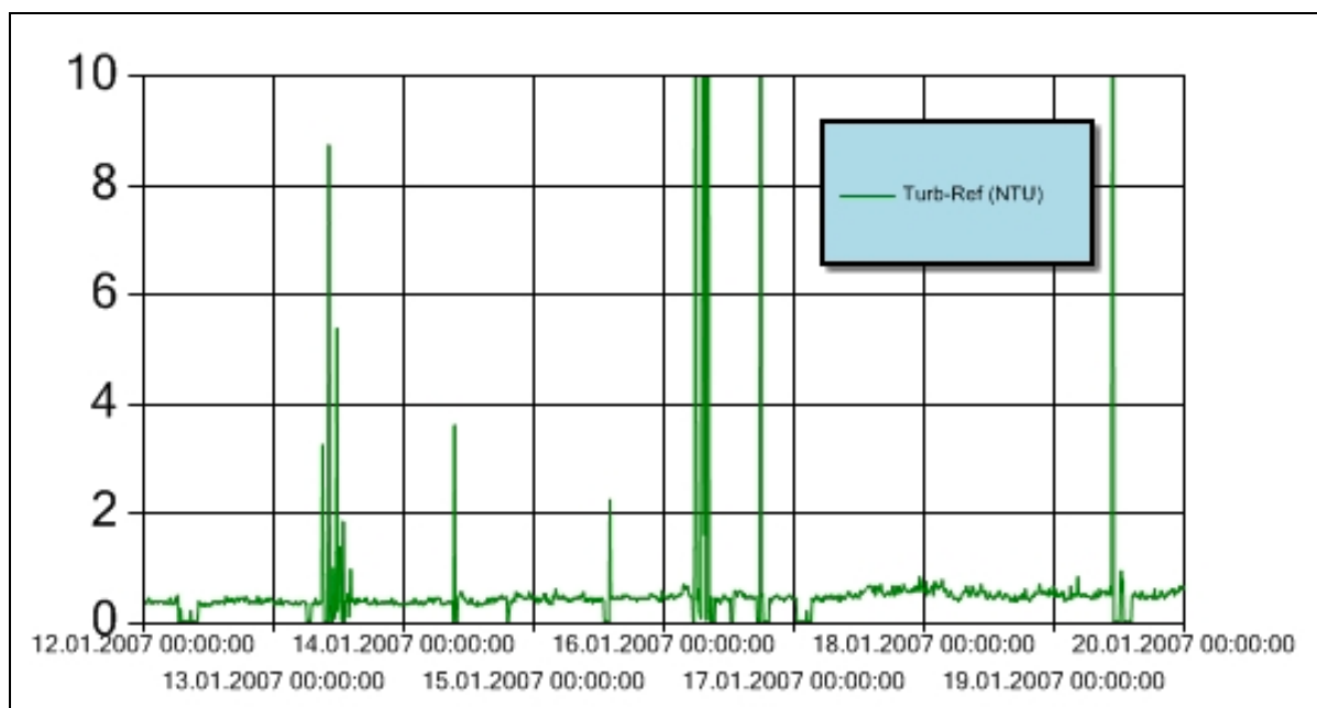
Figur 7 Turbiditet for perioden 12.-19. januar 2007 ved referansestasjonen i Bekkelagsbassenget. Turbiditetsensoren er plassert 3 m over sjøbunnen. Y-aksen angir målt turbiditet (NTU). Det er registrert episoder med signalstøy, enten i form av negative verdier eller unormalt høye verdier.
