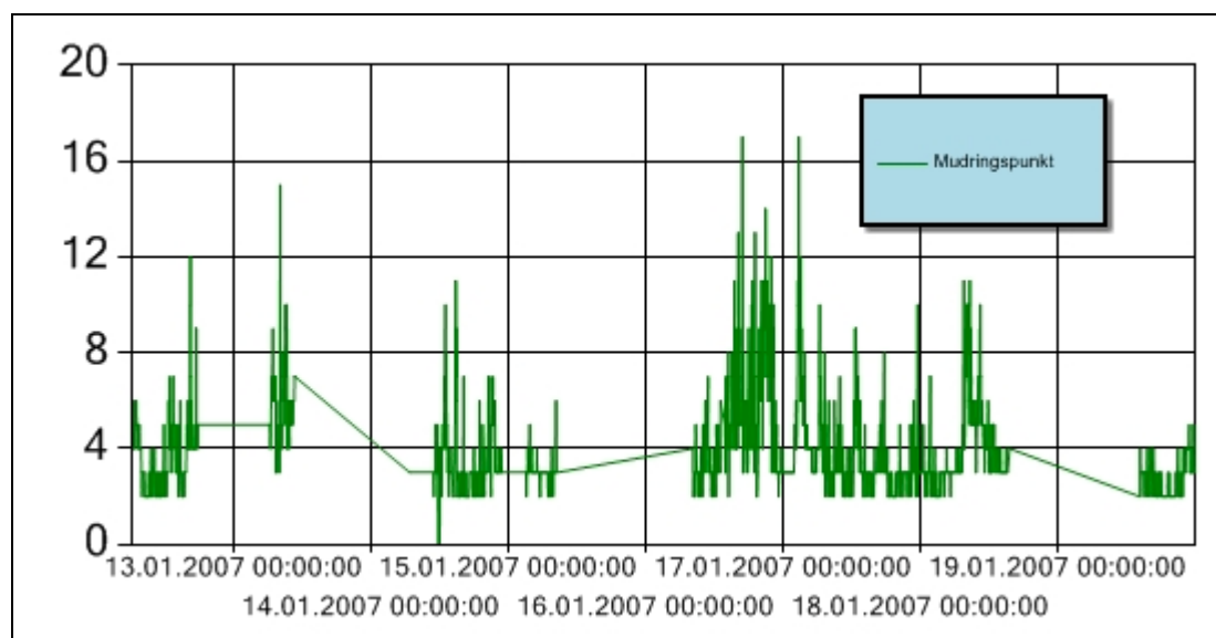
Figur 1 Turbiditet for perioden 12.-19. januar 2007 ved mudringslekker. Y-aksen angir målt turbiditet (NTU). Alle stopp som følge av overskredet grenseverdi for turbiditet blir dokumentert i månedsrapport for januar.
