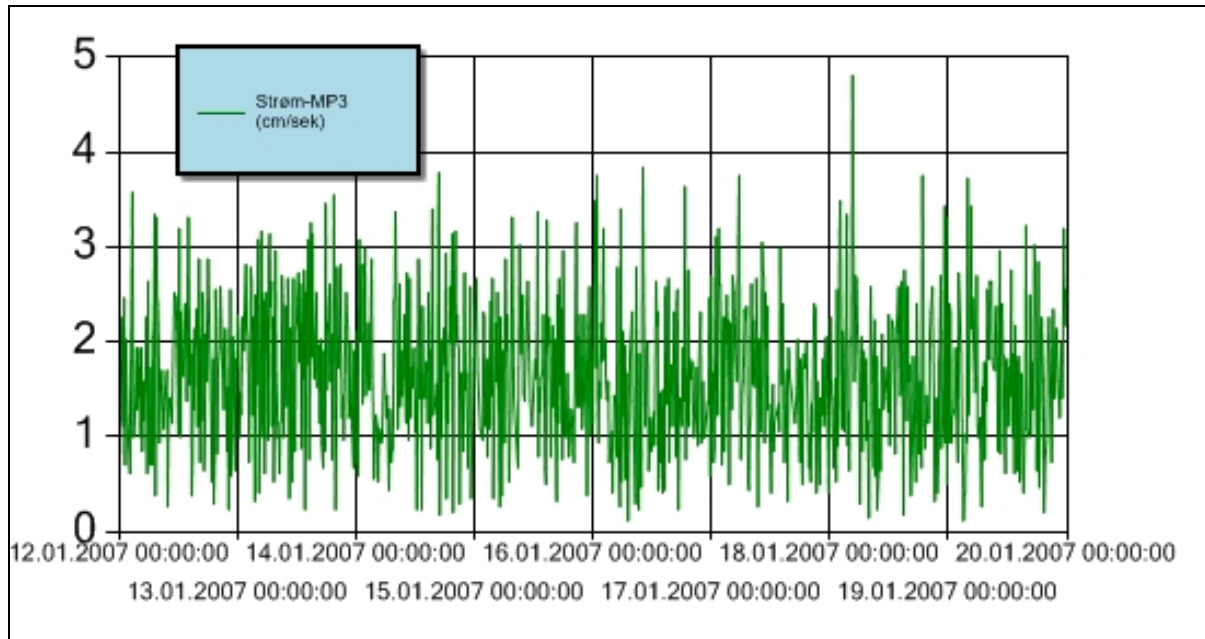
Figur 8 Strømhastighet for perioden 12.-19. januar 2007 ved målestasjon MP3. Y-aksen angir strømhastighet i cm/sekund. Sensoren er forankret slik at den henger fritt 3 m over sjøbunnen.
