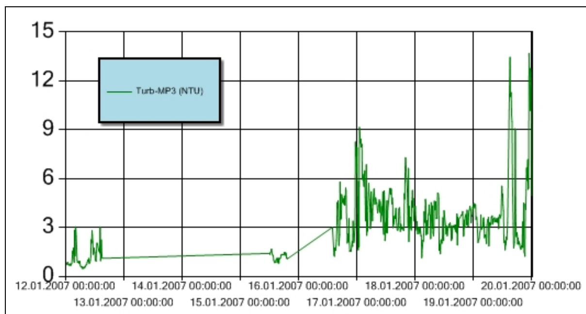
Figur 5 Turbiditet for perioden 12.-19. januar 2007 ved målestasjon MP3. Y-aksen angir målt turbiditet (NTU). Turbiditetsensoren er plassert 3 m over sjøbunnen. Det mangler data fra MP3 i perioden 12.-16. januar 2007. Disse dataene er forsøkt logget ned fra bøyens instrumentlogger, men dataene eksisterer ikke. Årsaken kan ha vært midlertidige problemer med strømforsyningen til sensoren. Ved MP3 er det registrert overskridelse av grenseverdien 19. januar 2007. Arbeidene ble stanset etter varsel via SMS.
