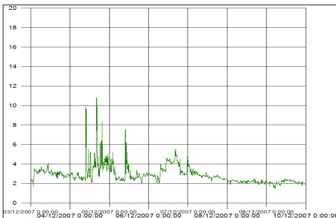
Figur 3 Turbiditet for perioden 3. – 9. desember 2007 ved mudringsleker i Bestumkilen. Y-aksen angir målt turbiditet (NTU). Alle stopp som følge av overskredet grenseverdi for turbiditet blir dokumentert i månedsrapport for desember.
