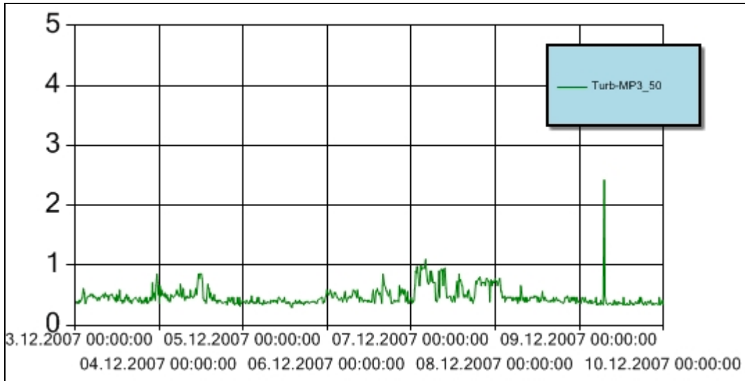
Figur 9 Turbiditet for perioden 3. – 9. desember 2007 ved målestasjon MP3_50. Y-aksen angir målt turbiditet (NTU). Turbiditetsensoren er plassert ved 50 m vanddyb. Høye enkeltmålinger skyldes støy.
