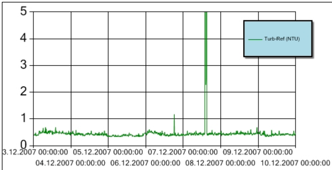
Figur 13 Turbiditet for perioden 3. – 9. desember 2007 ved referansestasjonen i Bekkelagsbassenget. Turbiditetsensoren er plassert ca. 3 m over sjøbunnen. Y-aksen angir målt turbiditet (NTU). Høye enkeltverdier skyldes støv.
