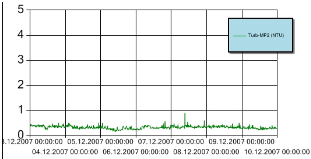
Figur 7 Turbiditet for perioden 3. – 9. desember 2007 ved målestasjon MP2. Y-aksen angir målt turbiditet (NTU). Turbiditetsensoren er plassert ca. 3 m over sjøbunnen.
