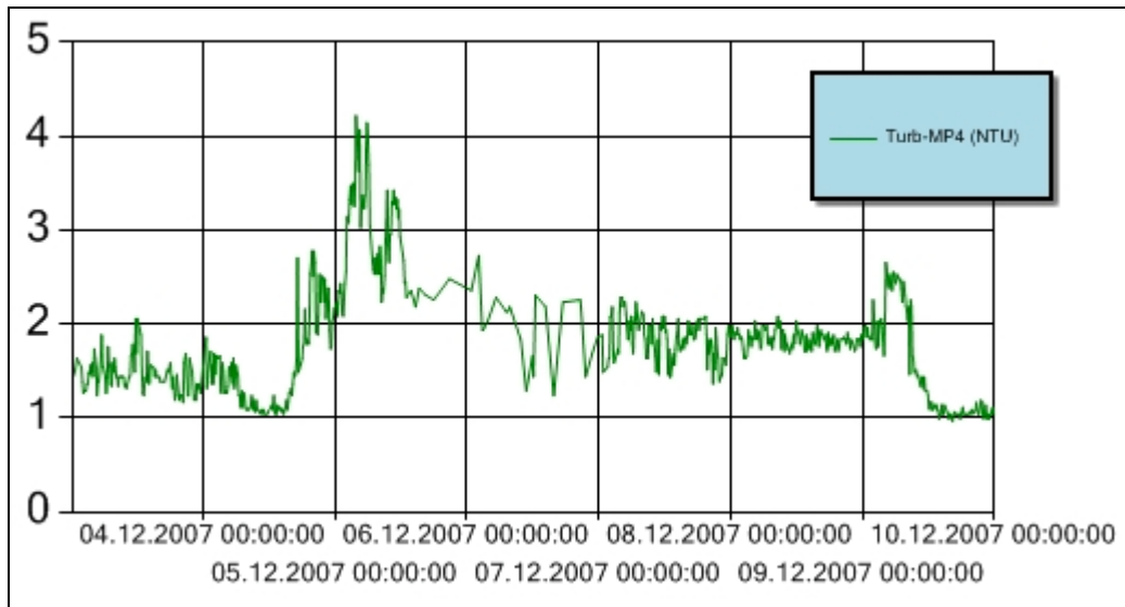
Figur 11 Turbiditet for perioden 3. – 9. desember ved målestasjon MP4. Y-aksen angir målt turbiditet (NTU). Turbiditetsensoren er plassert ca. 3 m over sjøbunnen.
