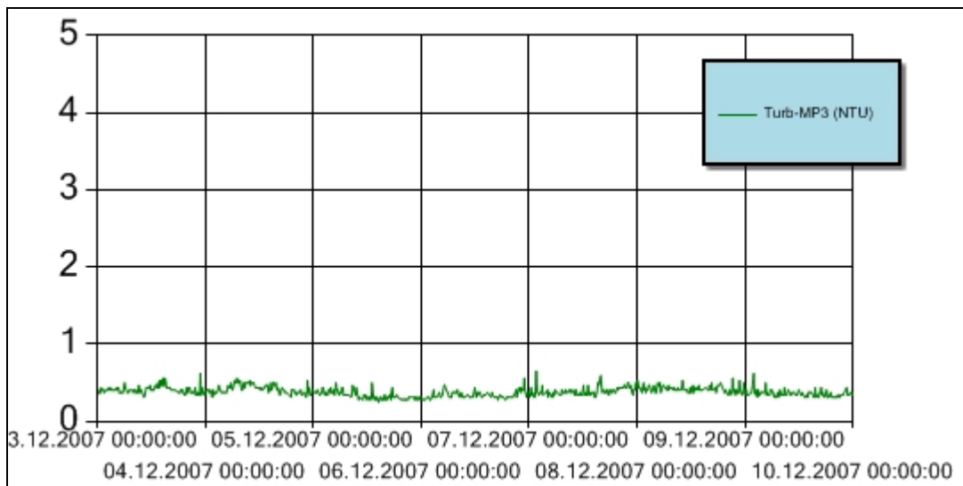
Figur 8 Turbiditet for perioden 3. – 9. desember 2007 ved målestasjon MP3. Y-aksen angir målt turbiditet (NTU). Turbiditetsensoren er plassert ca. 3 m over sjøbunnen.
