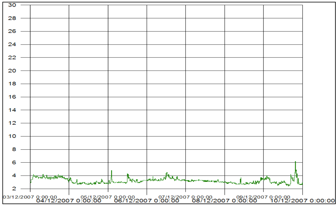
Figur 4 Turbiditet for perioden 3. – 9. desember 2007 ved referansestasjonen ved serviceflåten i Bestumkilen under mudring i Bestumkilen. Y-aksen angir målt turbiditet (NTU).
