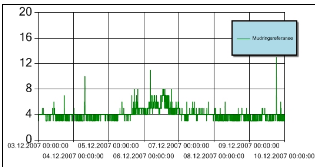
Figur 2 Turbiditet for perioden 3. – 9. desember 2007 ved referansestasjonen ved Akershusutstikkeren under mudring i Pipervika. Y-aksen angir målt turbiditet (NTU).
