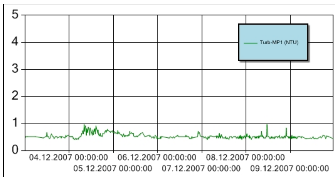
Figur 6 Turbiditet for perioden 3. – 9. desember 2007 ved målestasjon MP1. Y-aksen angir målt turbiditet (NTU). Turbiditetsensoren er plassert ca. 3 m over sjøbunnen.
