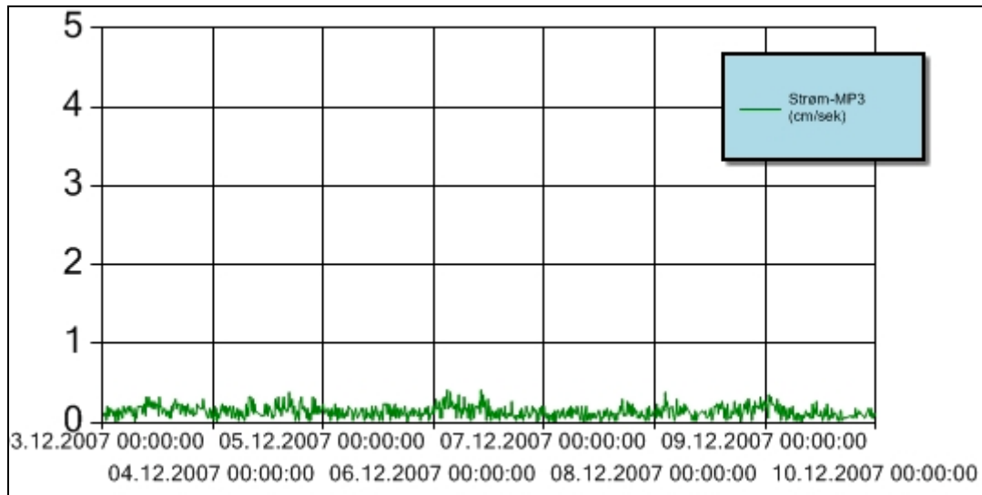
Figur 15 Strømhastighet for perioden 3. – 9. desember 2007 ved målestasjon MP3. Y-aksen angir strømhastighet i cm/sekund. Sensoren er forankret slik at den henger fritt ca. 3 m over sjøbunnen.
