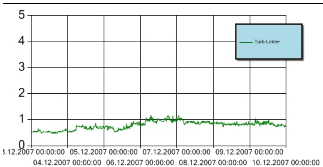
Figur 14 Turbiditet for perioden 3. – 9. desember 2007 ved H2, nedføringsenheten. Turbiditetsensoren er plassert ca. 10 m under overflata. Y-aksen angir målt turbiditet (NTU).
