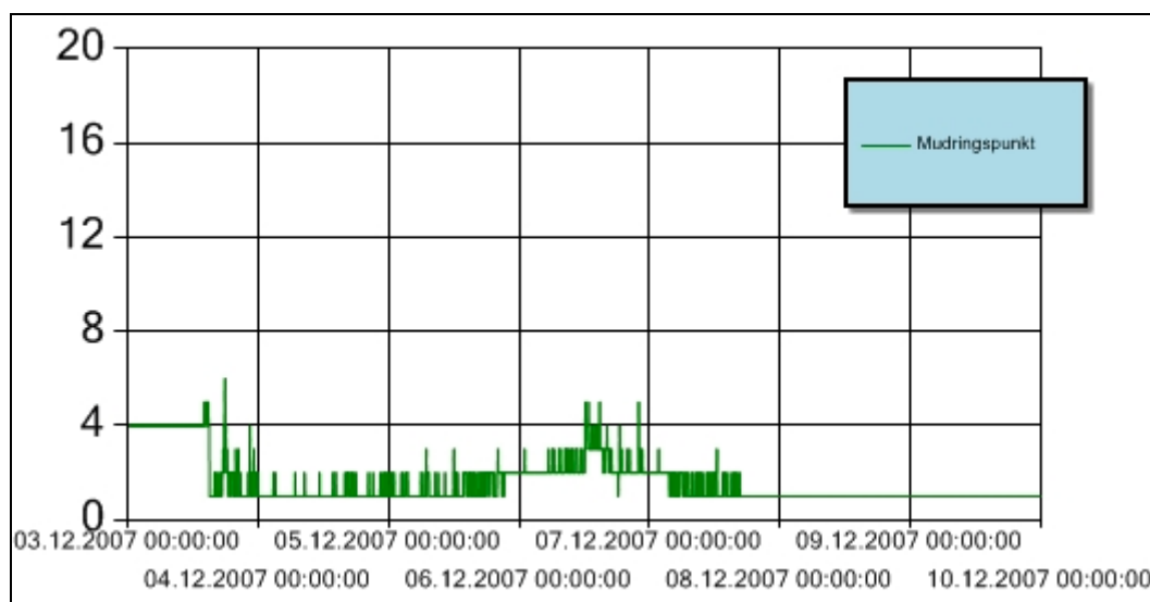
Figur 1 Turbiditet for perioden 3. – 9. desember 2007 ved mudringslekter under mudring i Pipervika. Y-aksen angir målt turbiditet (NTU). Alle stopp som følge av overskredet grenseverdi for turbiditet blir dokumentert i månedsrapport for desember.
