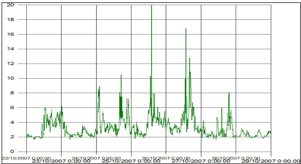
Figur 3 Turbiditet for perioden 22. – 28. oktober 2007 ved mudringslekter i Bestumkilen. Y-aksen angir målt turbiditet (NTU). Alle stopp som følge av overskredet grenseverdi for turbiditet blir dokumentert i månedsrapport for oktober.
