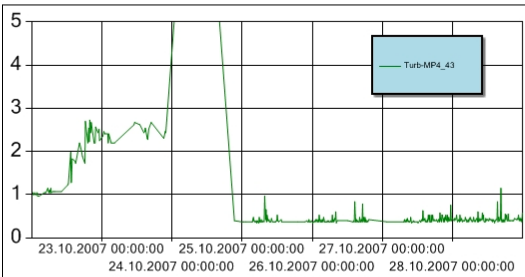
Figur 12 Turbiditet for perioden 22. – 28. oktober 2007 ved målestasjon MP4_43. Y-aksen angir målt turbiditet (NTU). Turbiditetsensoren er plassert ved 43 m vann dybde. Bøyen slet seg fra festet i uke 40, og har vært forankret i MP1 til den 24. oktober. Data fra før 24. oktober blir ikke benyttet i statistiske beregninger.
