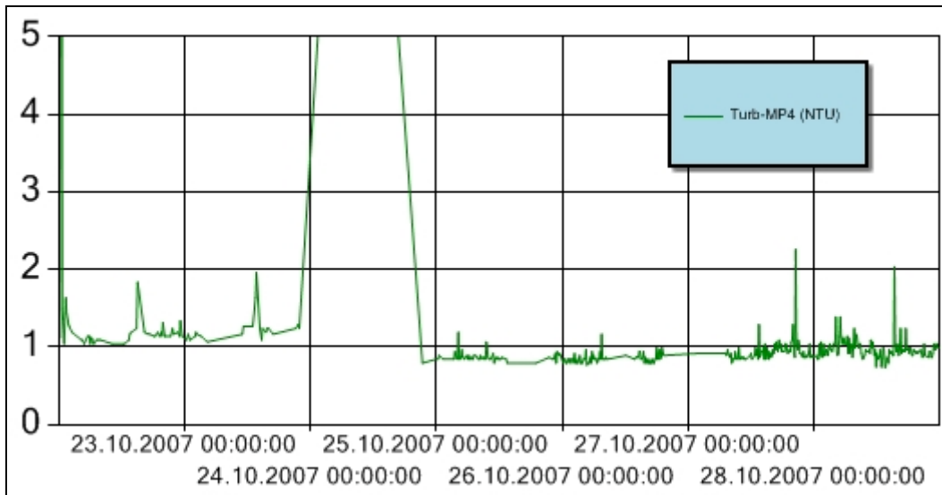
Figur 11 Turbiditet for perioden 22. – 28. oktober 2007 ved målestasjon MP4. Y-aksen angir målt turbiditet (NTU). Turbiditetsensoren er plassert ca. 3 m over sjøbunnen. Bøyen slet seg fra festet i uke 40, og har vært forankret i MP1 til den 24. oktober. Data fra før 24. oktober blir ikke benyttet i statistiske beregninger, fordi bøyen ligger fortøyd i MP1 og den nederste måleren ligger på bunnen.
