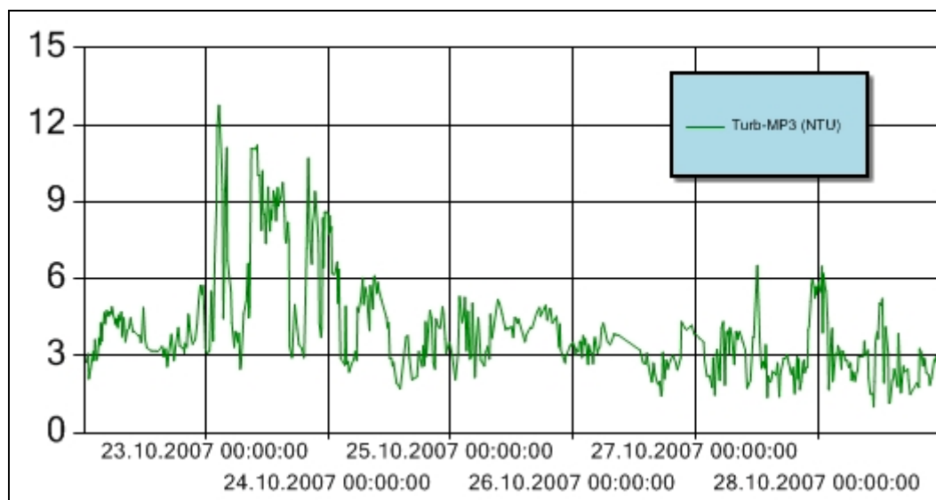
Figur 8 Turbiditet for perioden 22. – 28. oktober 2007 ved målestasjon MP3. Y-aksen angir målt turbiditet (NTU). Turbiditetsensoren er plassert ca. 3 m over sjøbunnen. Merk at MP3 er oppgitt med en annen skala enn de andre målerne.
