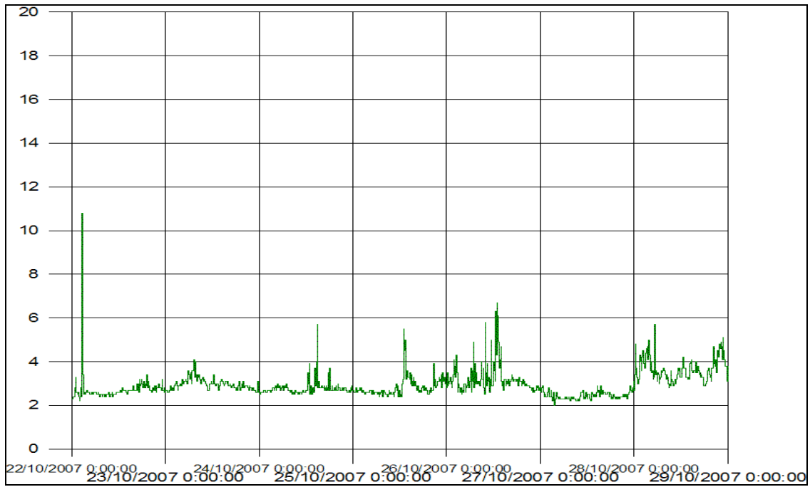
Figur 4 Turbiditet for perioden 22. – 28. oktober 2007 ved referansestasjonen ved serviceflåten i Bestumkilen under mudring i Bestumkilen. Y-aksen angir målt turbiditet (NTU). Høye enkeltmålinger skyldes støy.
