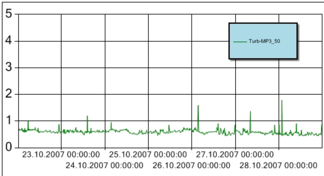
Figur 9 Turbiditet for perioden 22. – 28. oktober 2007 ved målestasjon MP3_50. Y-aksen angir målt turbiditet (NTU). Turbiditetsensoren er plassert ved 50 m vanddyb.
