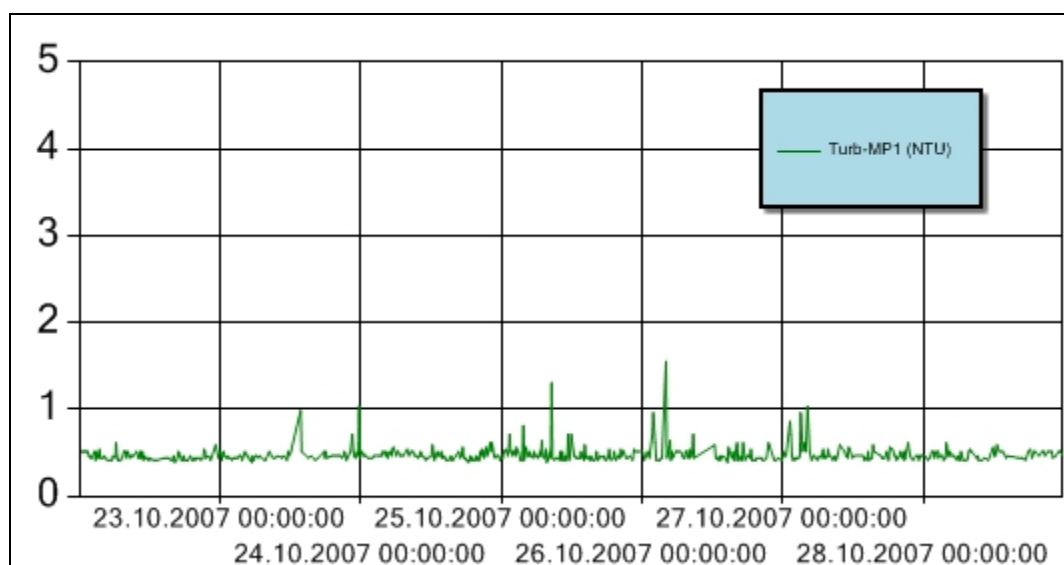
Figur 6 Turbiditet for perioden 22. – 28. oktober 2007 ved målestasjon MP1. Y-aksen angir målt turbiditet (NTU). Turbiditetsensoren er plassert ca. 3 m over sjøbunnen.
