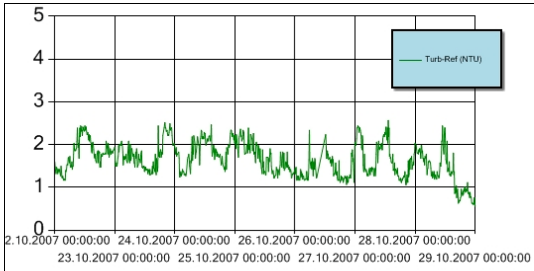
Figur 13 Turbiditet for perioden 22. – 28. oktober 2007 ved referansestasjonen i Bekkelagsbassenget. Turbiditetsensoren er plassert ca. 3 m over sjøbunnen. Y-aksen angir målt turbiditet (NTU).
