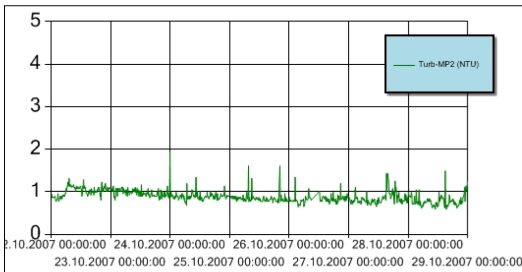
Figur 7 Turbiditet for perioden 22. – 28. oktober 2007 ved målestasjon MP2. Y-aksen angir målt turbiditet (NTU). Turbiditetsensoren er plassert ca. 3 m over sjøbunnen.
