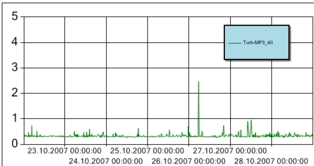
Figur 10 Turbiditet for perioden 22. – 28. oktober 2007 ved målestasjon MP3_40. Y-aksen angir målt turbiditet (NTU). Turbiditetsensoren er plassert ved 40 m vanddyb.
