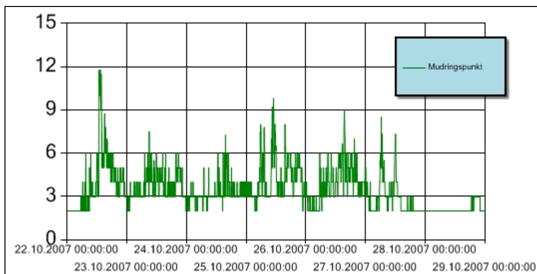
Figur 1 Turbiditet for perioden 22. – 28. oktober 2007 ved mudringslekter under mudring i Lohavn. Y-aksen angir målt turbiditet (NTU). Alle stopp som følge av overskredet grenseverdi for turbiditet blir dokumentert i månedsrapport for oktober.
