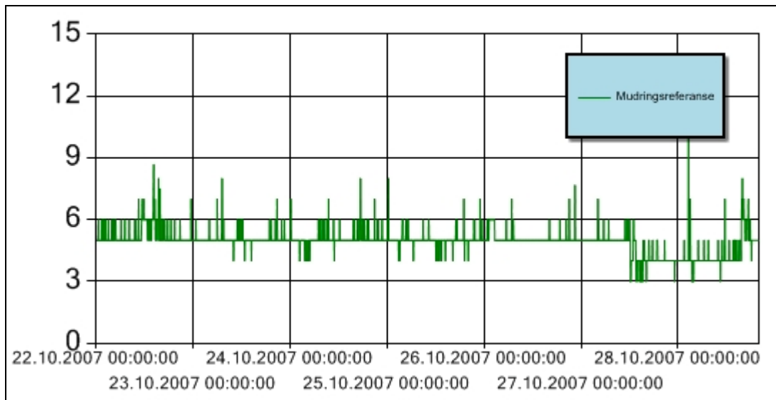
Figur 2 Turbiditet for perioden 22. – 28. oktober 2007 ved referansestasjonen ved Sørengutstikkeren under mudring i Lohavn. Y-aksen angir målt turbiditet (NTU). Høye enkeltmålinger skyldes støv.
